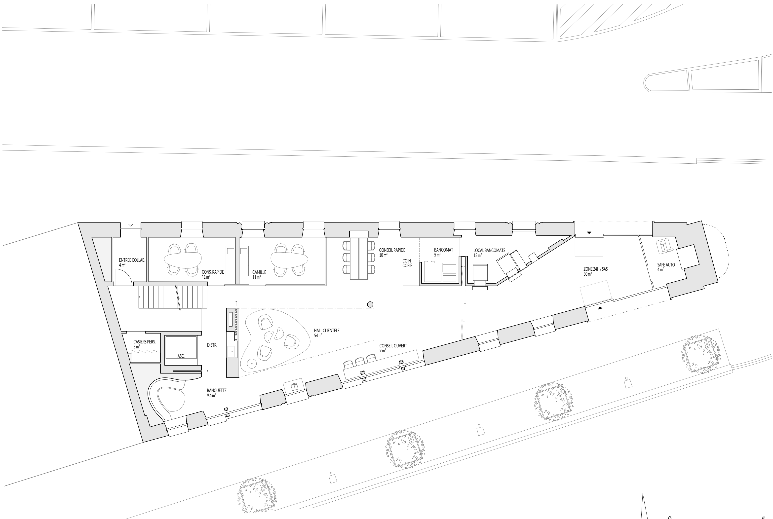
PLAN DE REZ-DE-CHAUSSEE BANQUE RAIFFEISEN DELEMONT - BURRI ET PARTENAIRES SARL - SEPTEMBRE 2020
