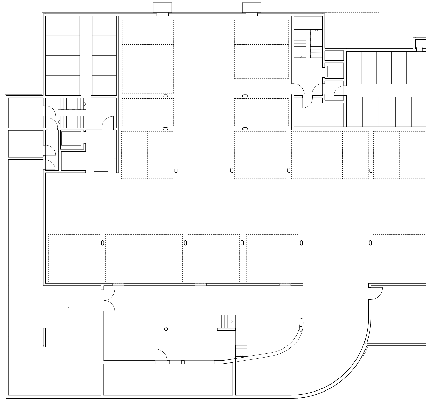
Untergeschoss 1:200
