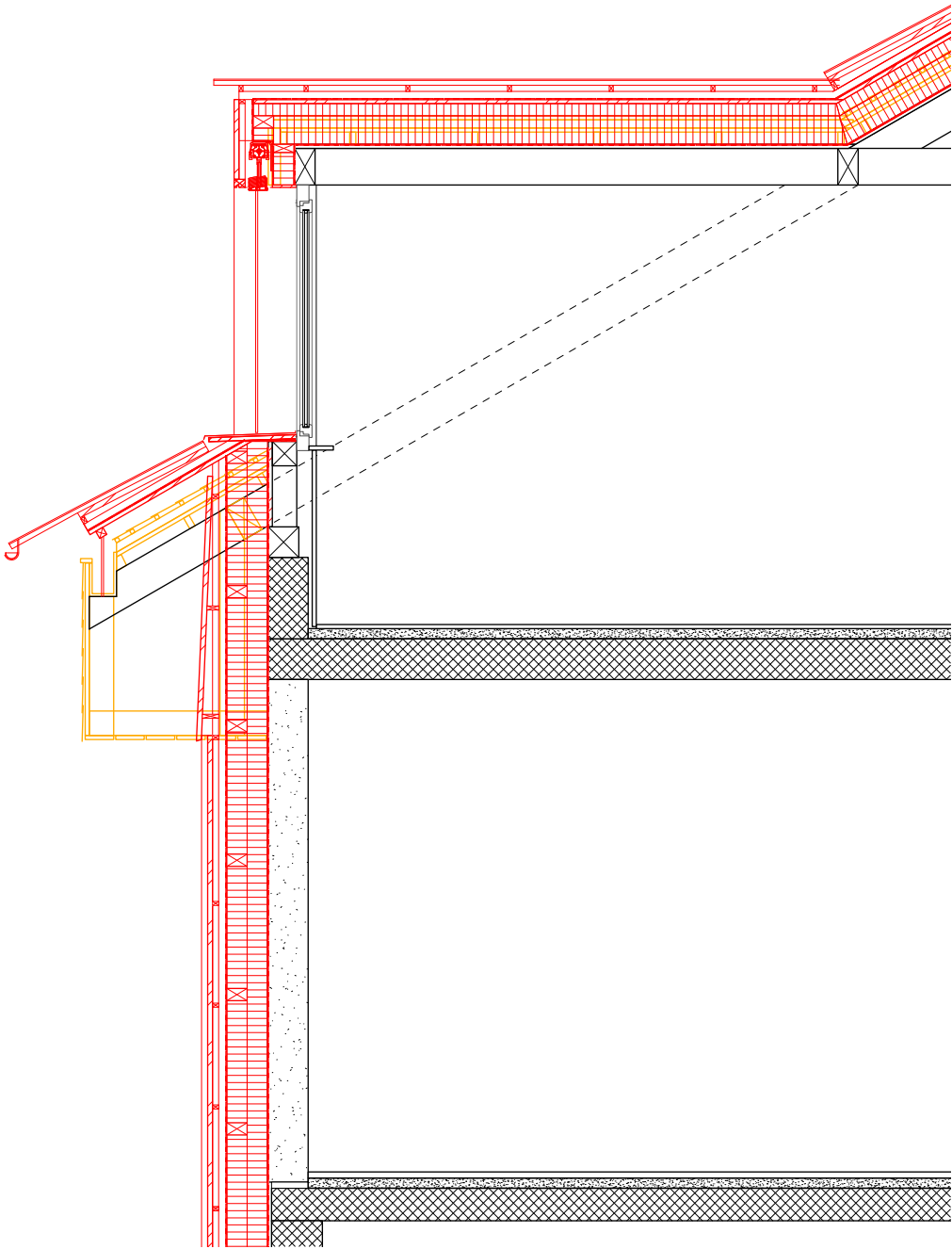
Detailschnitt Gaube
