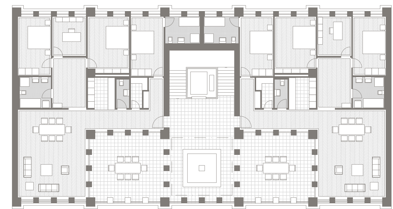
grundriss niveau 03_06_09 1_200
