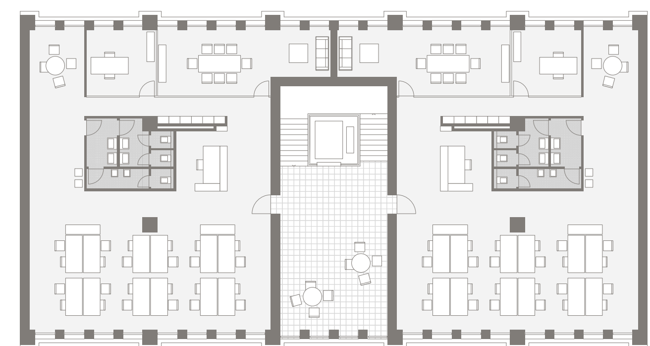
grundriss niveau 02 1_200
