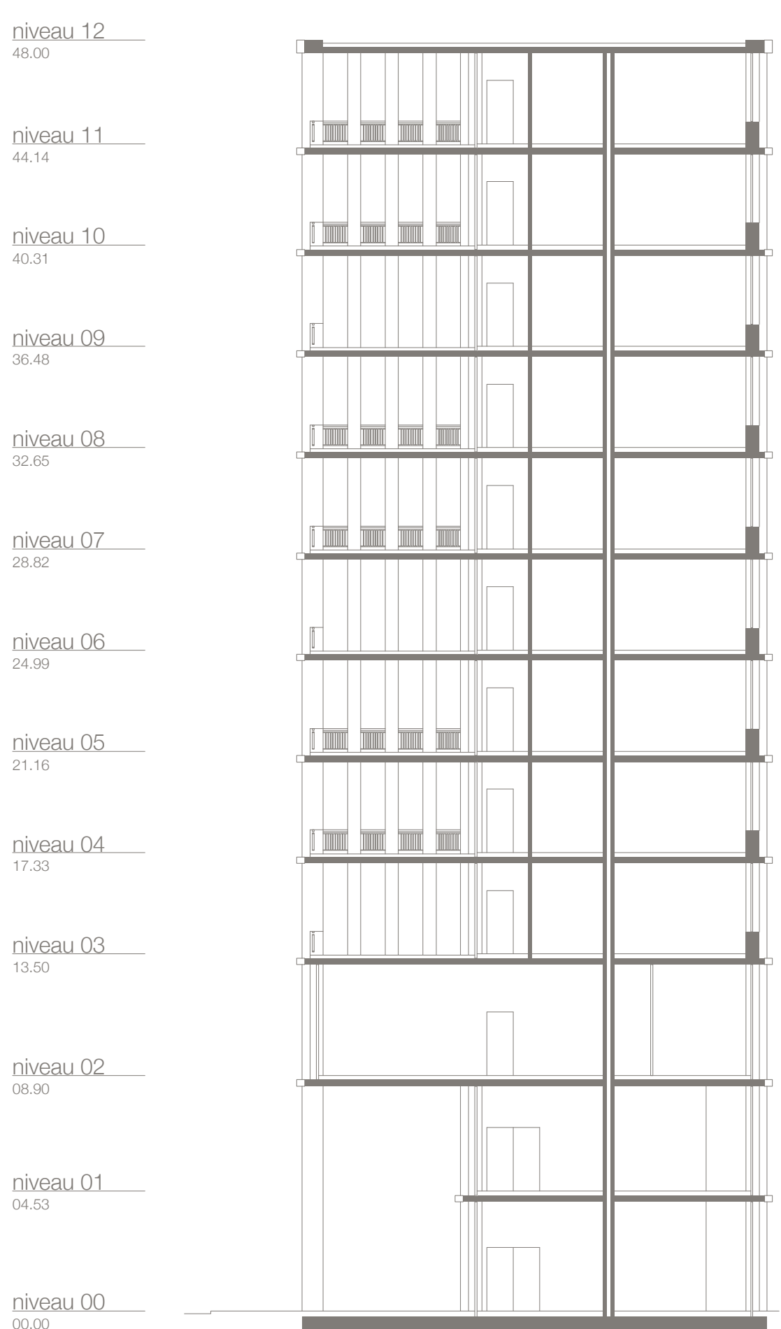
querschnitt 1_200
