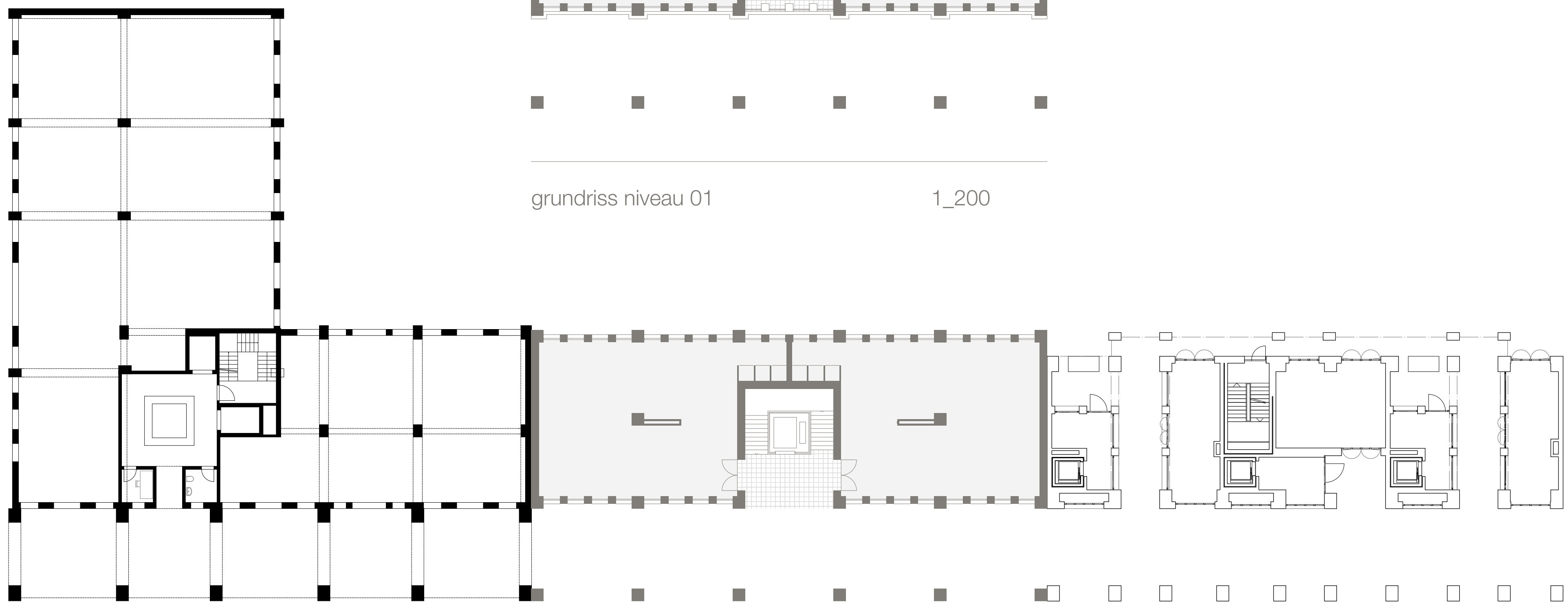
grundriss niveau 00 1_200
