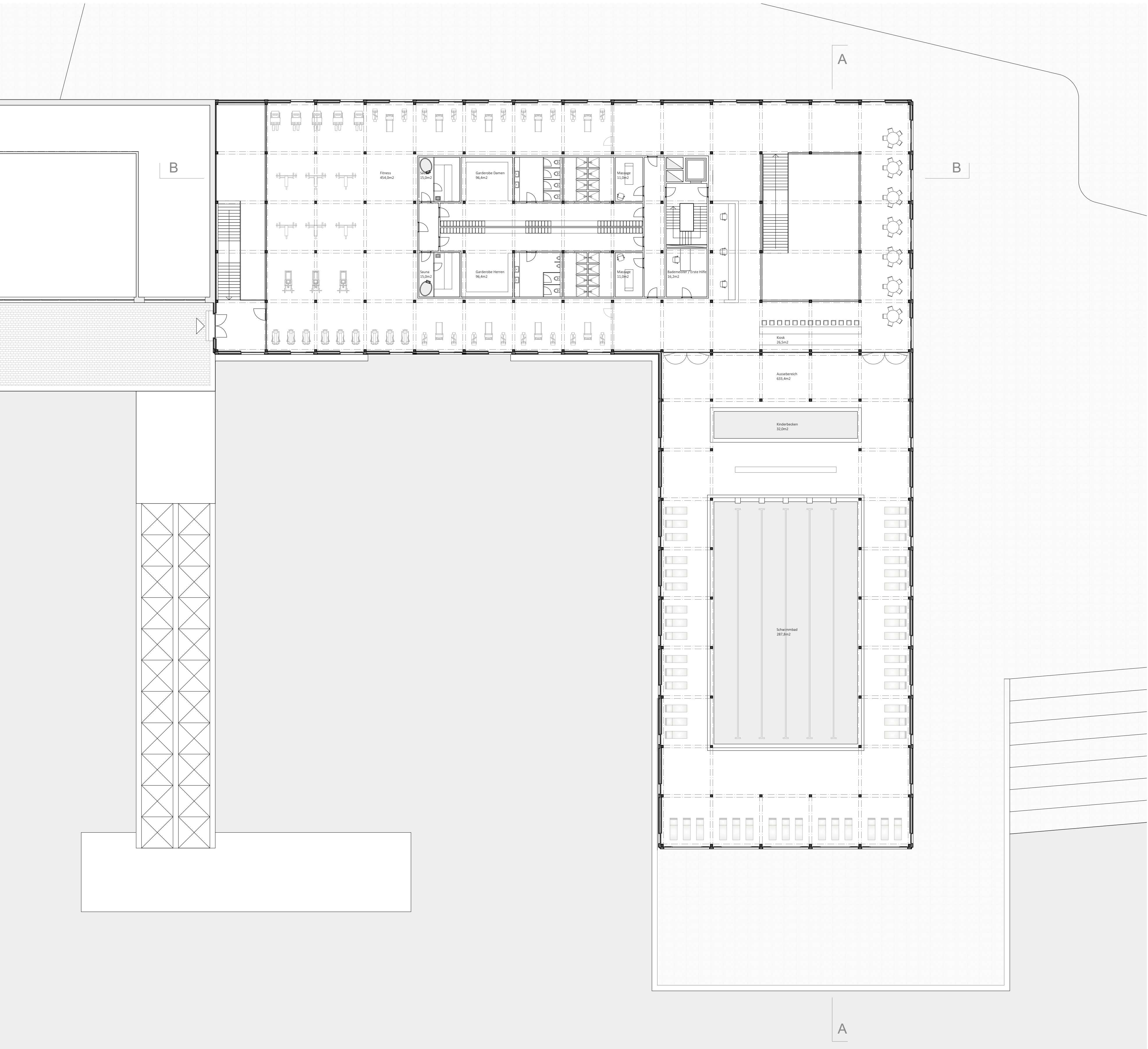
Grundriss 1. Obergeschoss Mst. 1:200
