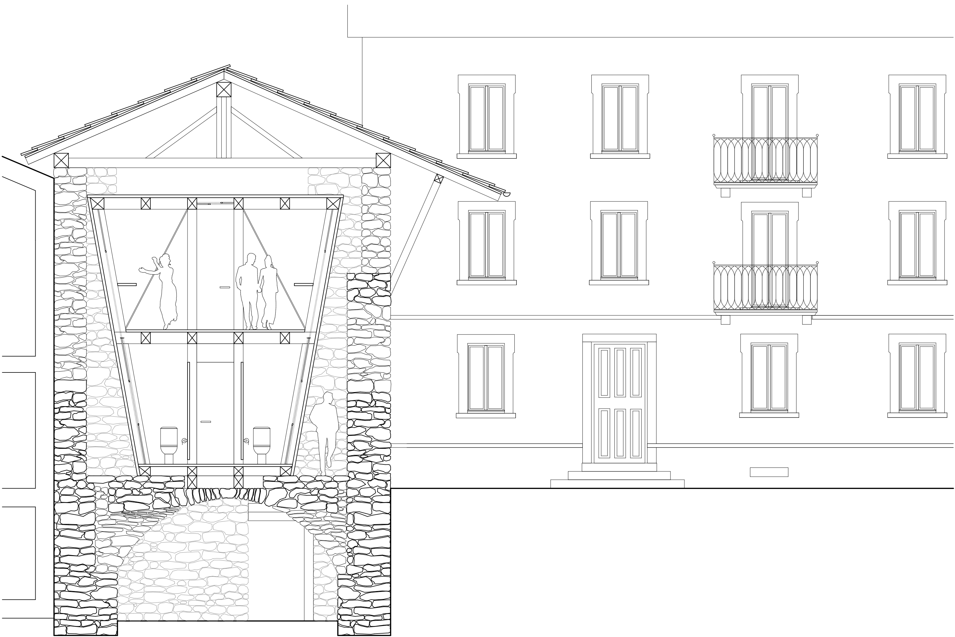
QUERSCHNITT 1:50
