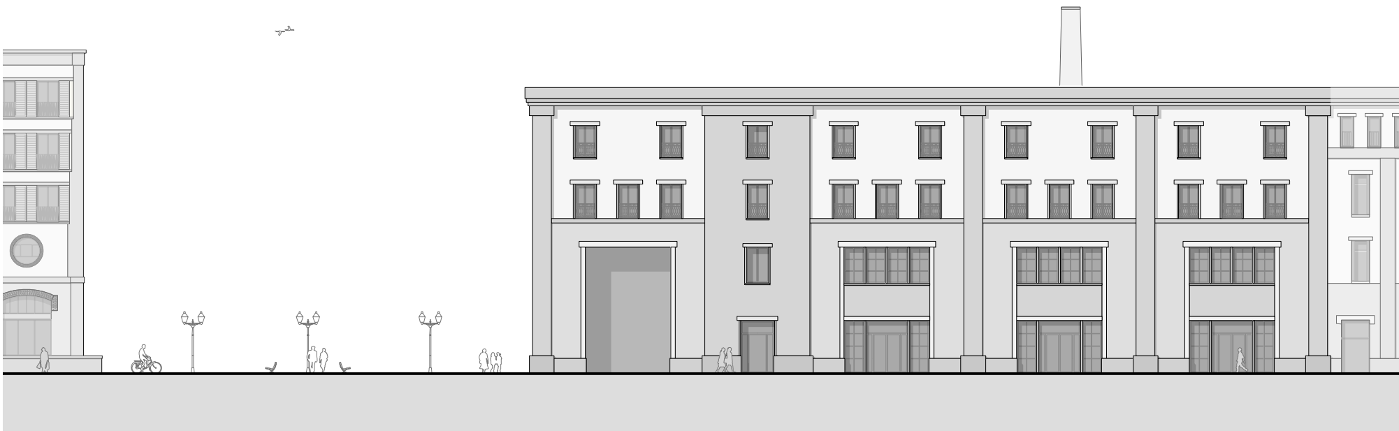
Ostfassade
