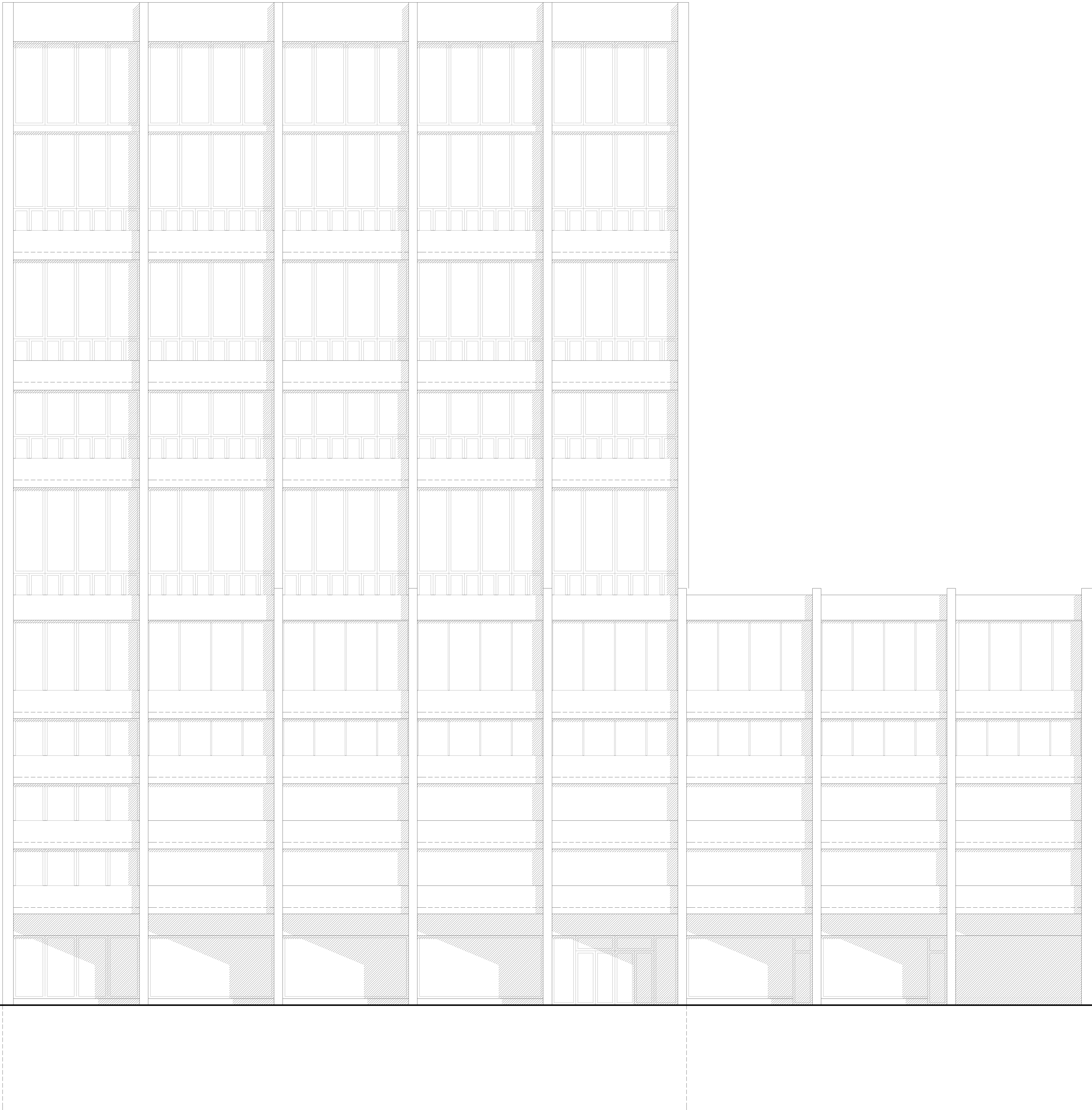
Ansicht Strassenfassade, Norden 1:100
