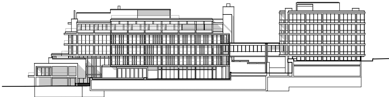
Südostansicht M1:700
