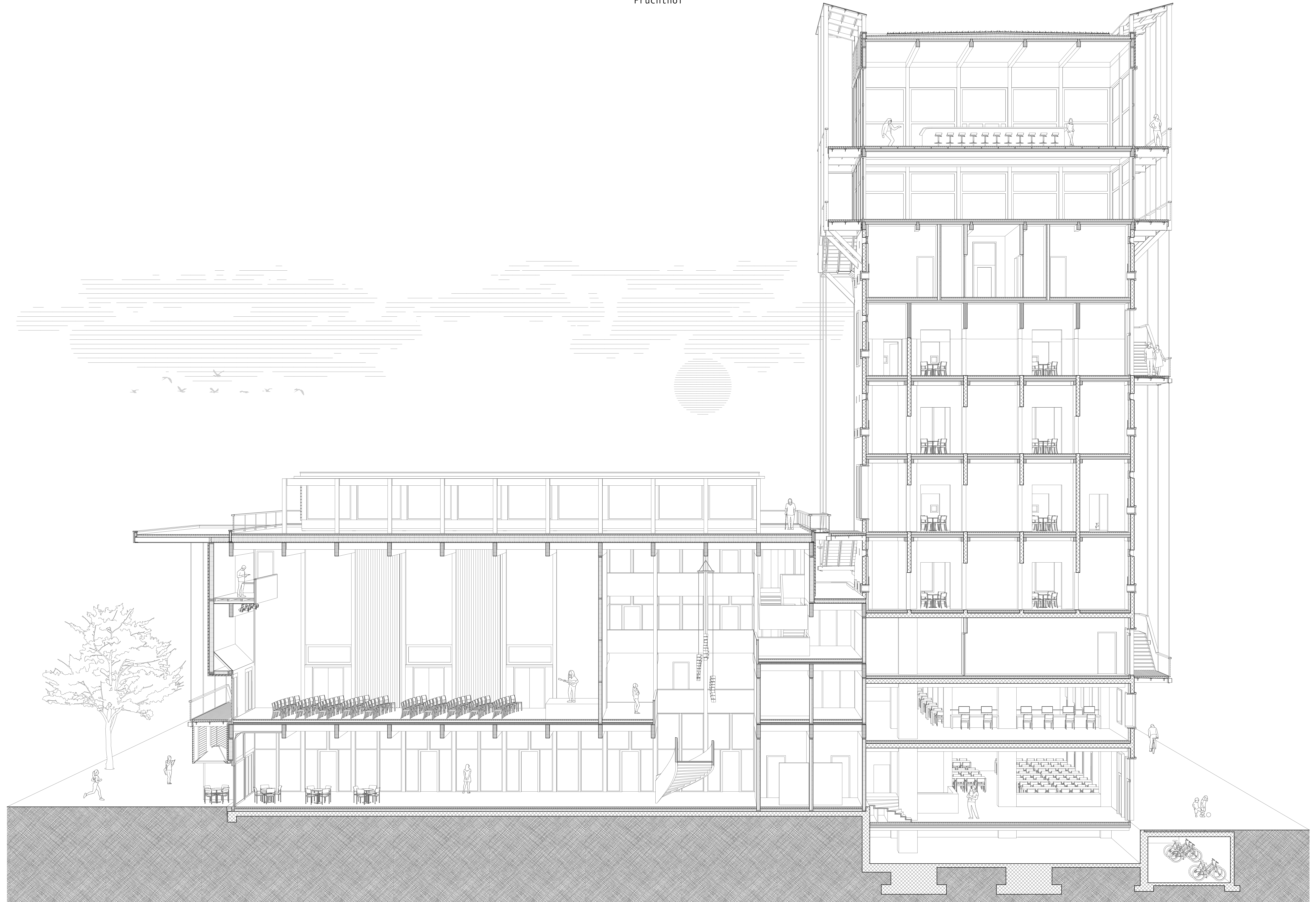
Hauptschnitt 1_66
