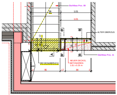
GRUNDRISS - EBENE 2
