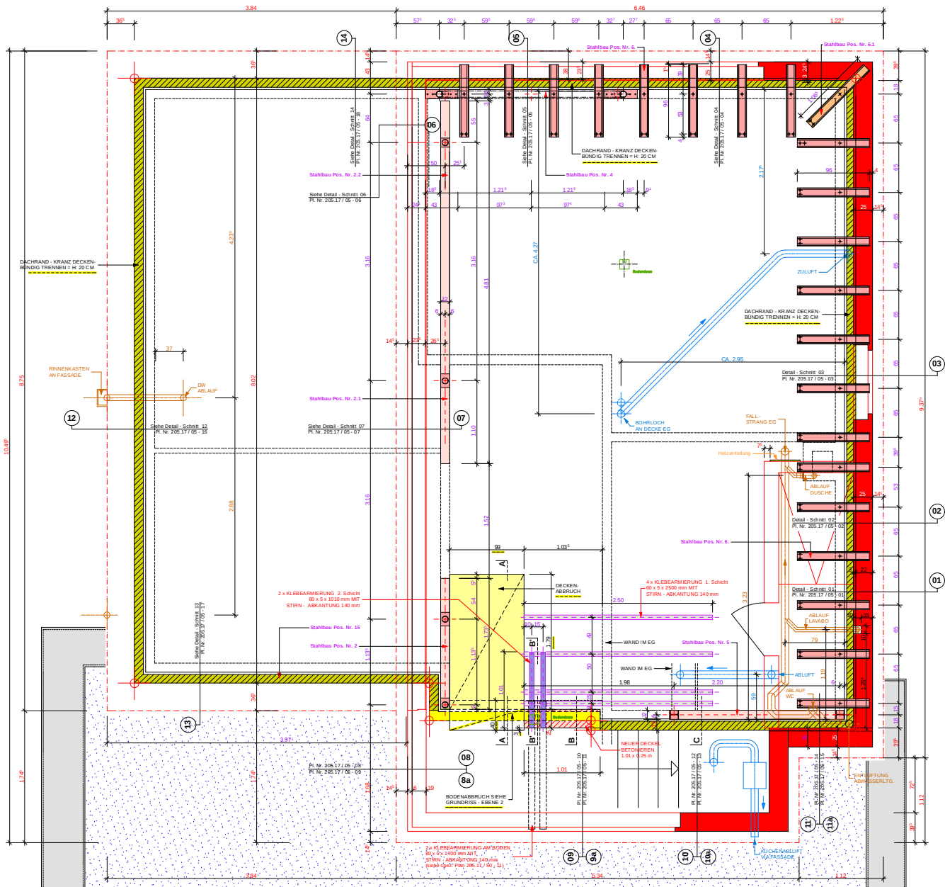
GRUNDRISS - EBENE 2
