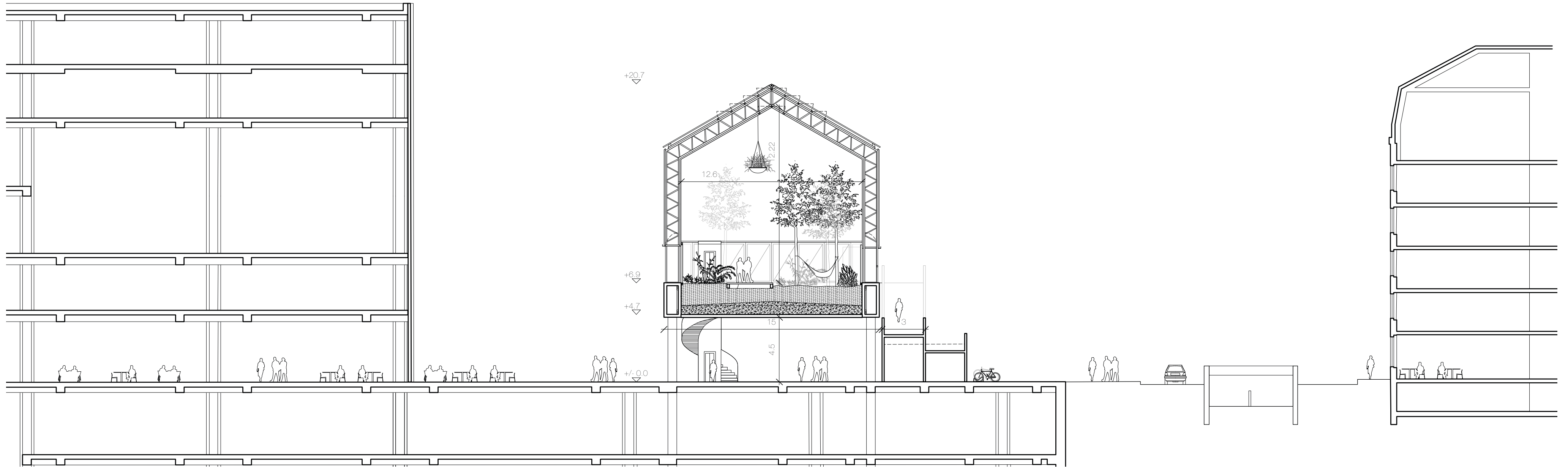
1:200 Schnitt 1-1
