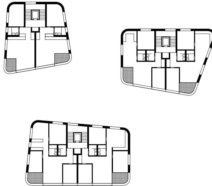
Grundriss OG
