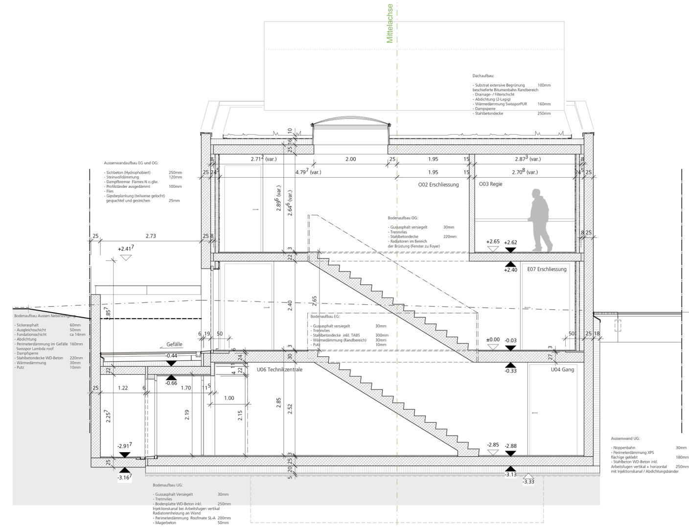
Querschnitt 3
