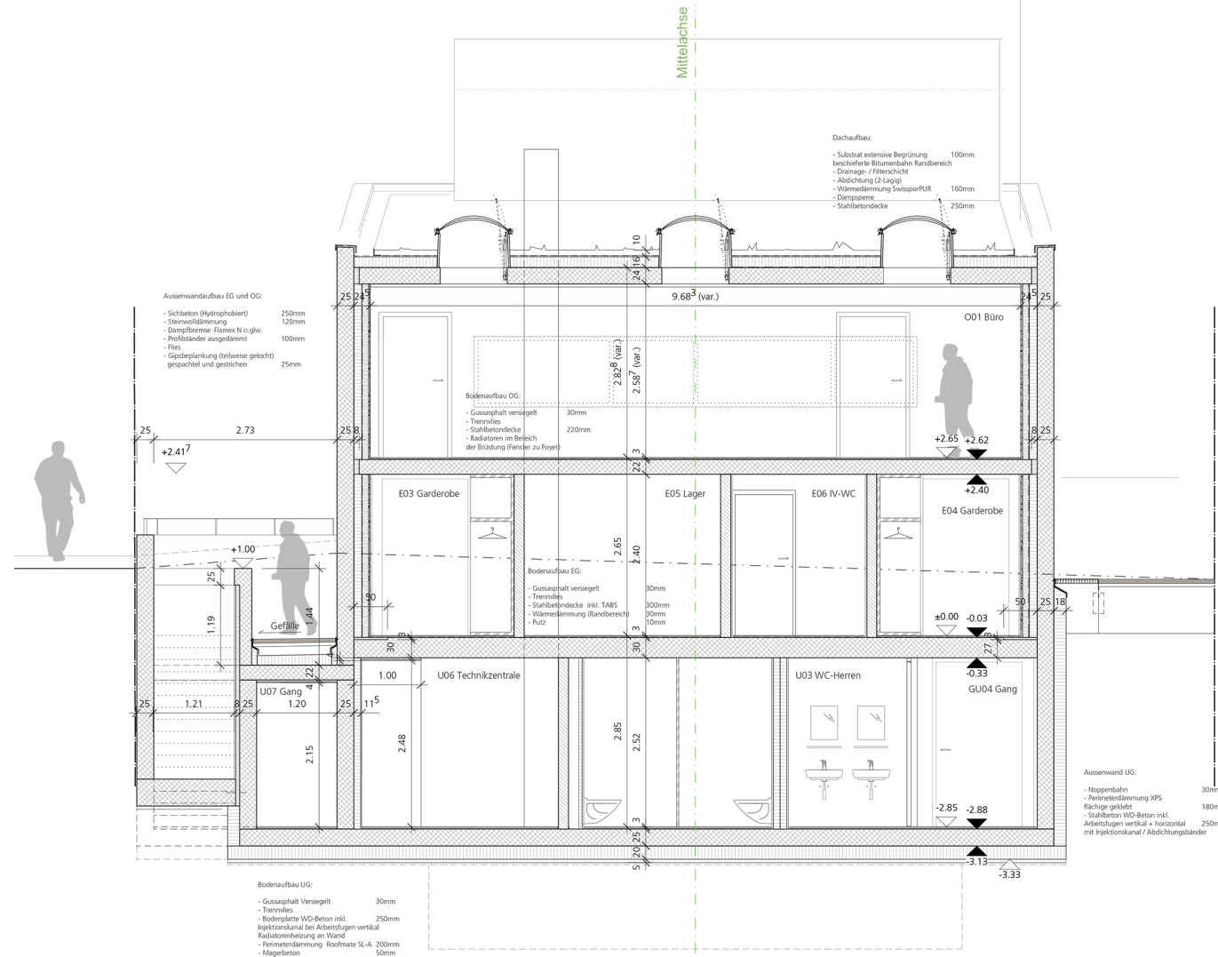
Querschnitt 2
