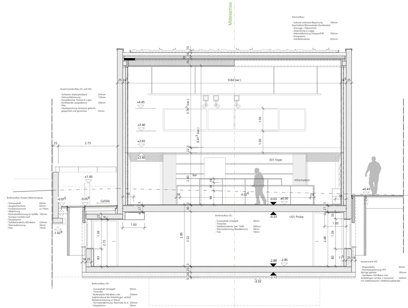
Querschnitt 1
