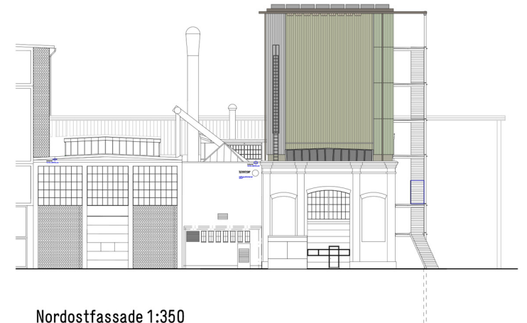
Nordostfassade 1:350
