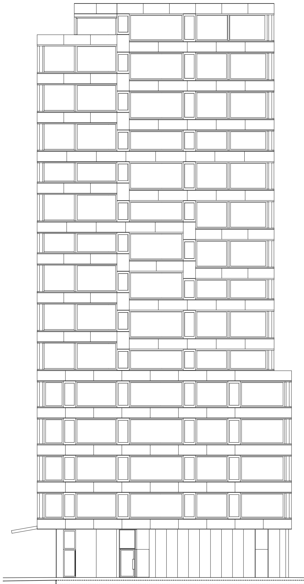
Ansicht OST Zeichnungsmaßstab 1:200
