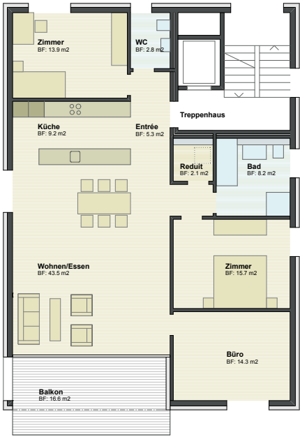
Wohnung 2 4 1/2 Zi Wohnung 121.0 m 2
