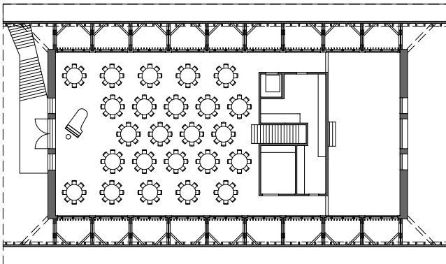
Grundriss Obergeschoss
