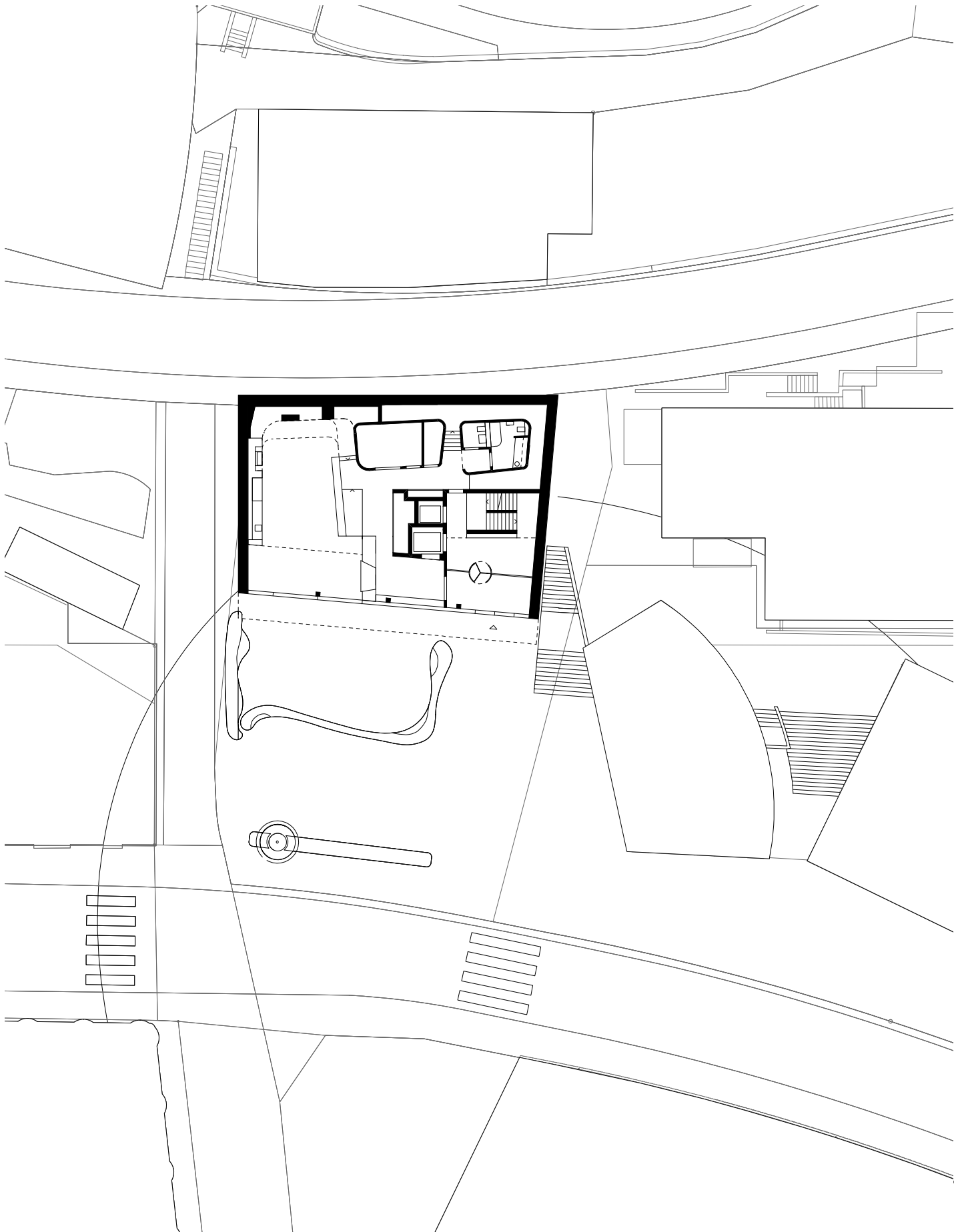
Erdgeschoss. Kinderkrippe
