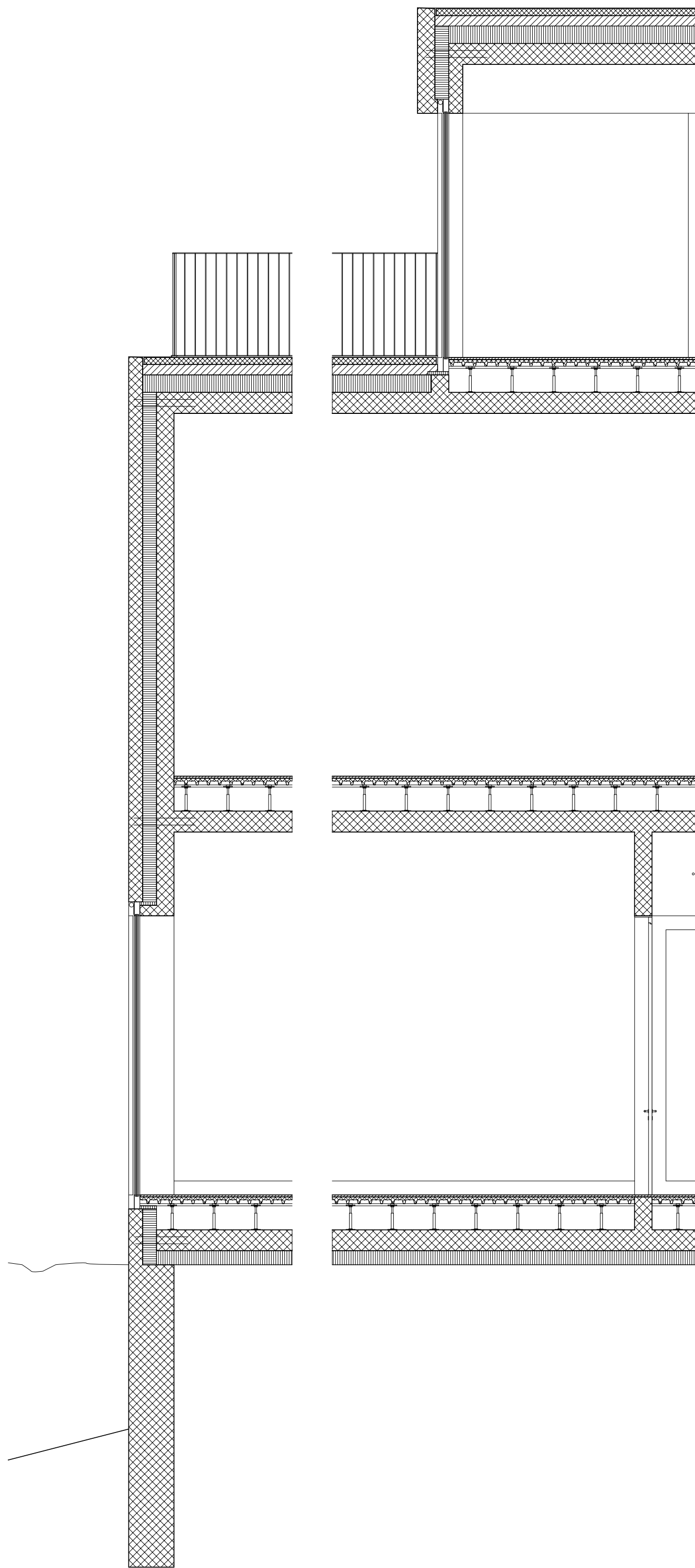
Coupe constructive | 1:50
