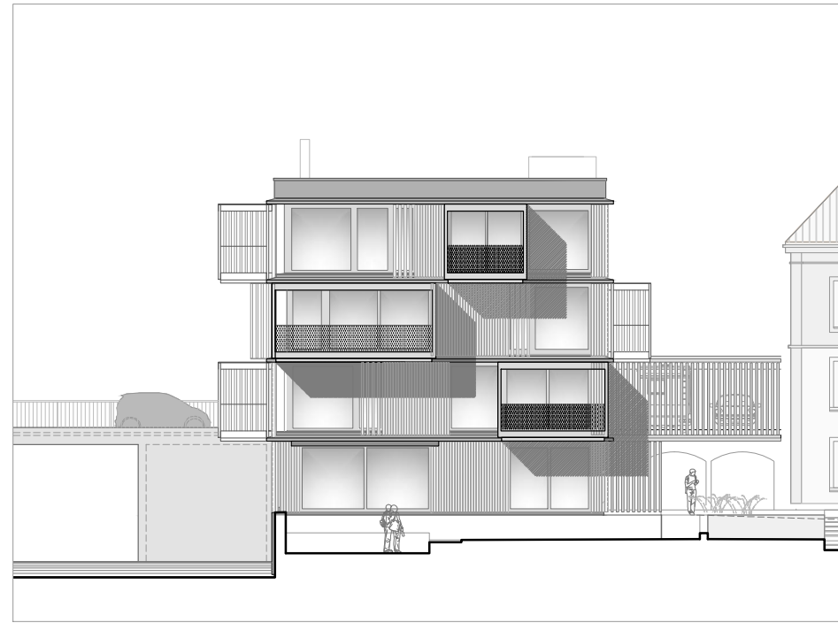
südfassade
