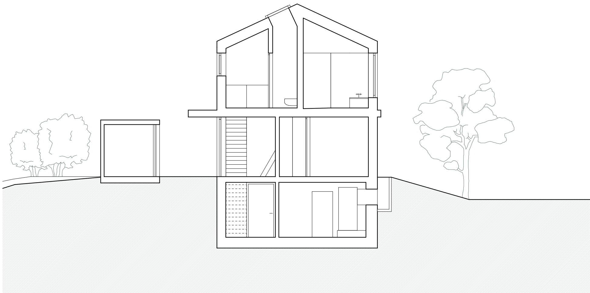
QUERSCHNITT 3
