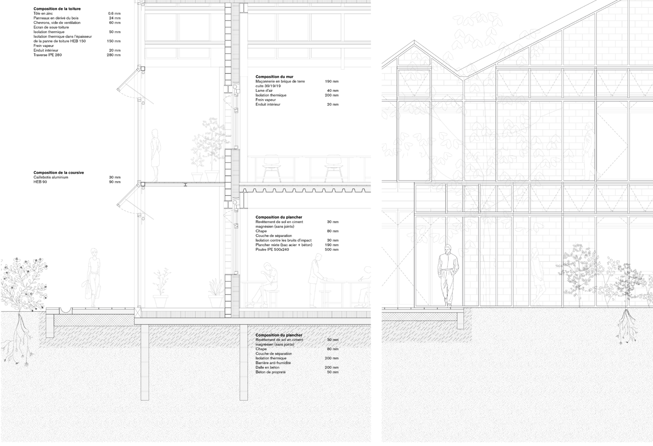
Coupe et façade détaillées 0 2 4 6 8 10m
