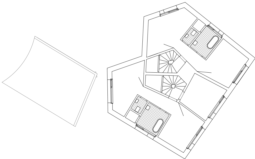
Obergeschoss 1:200
