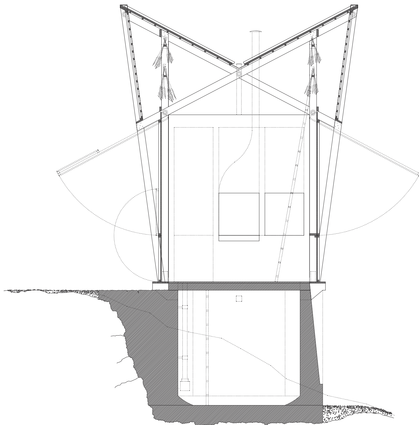
Coupe transversale AA' - échelle 1.50 -
