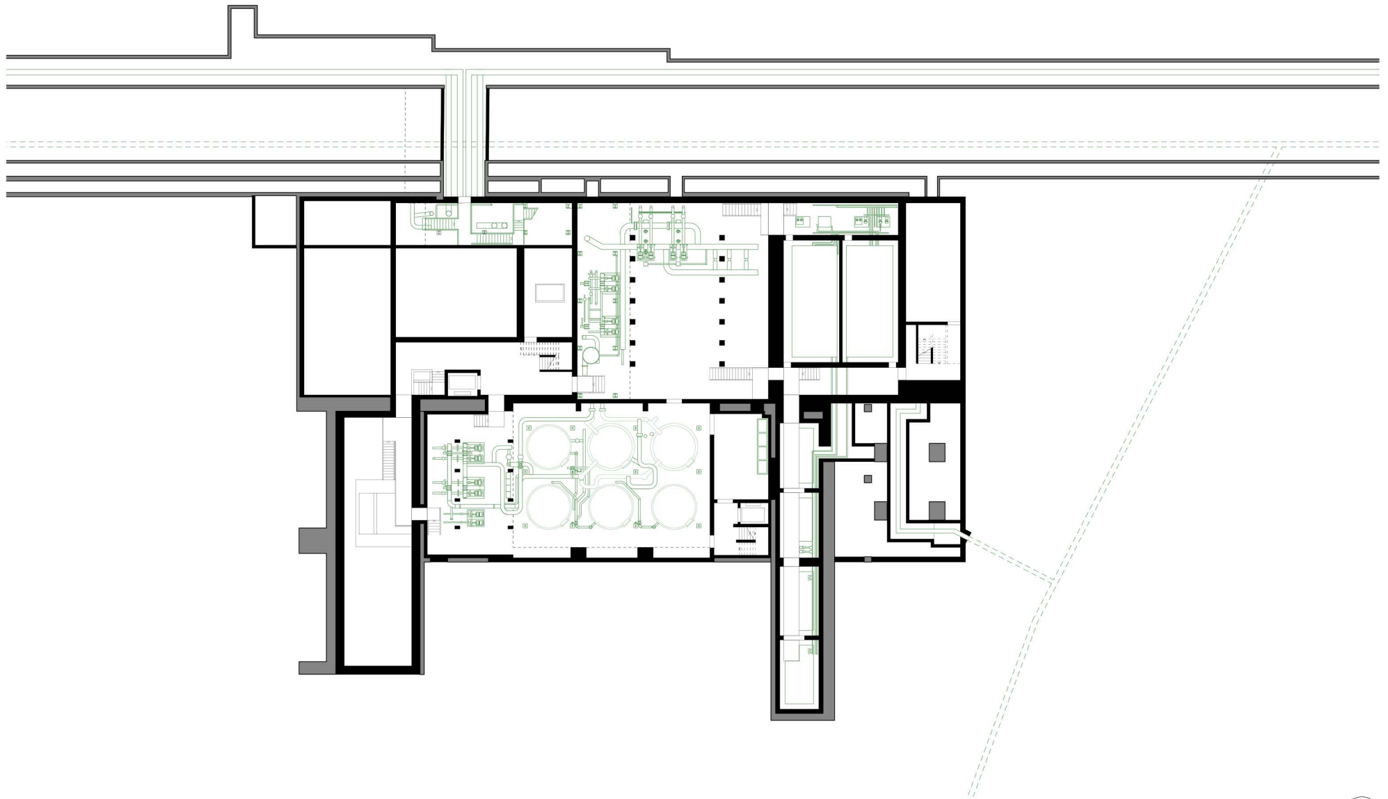
Grundriss 1. Untergeschoss, WZW Energiezentrale Josefstrasse, Zürich 1:500
