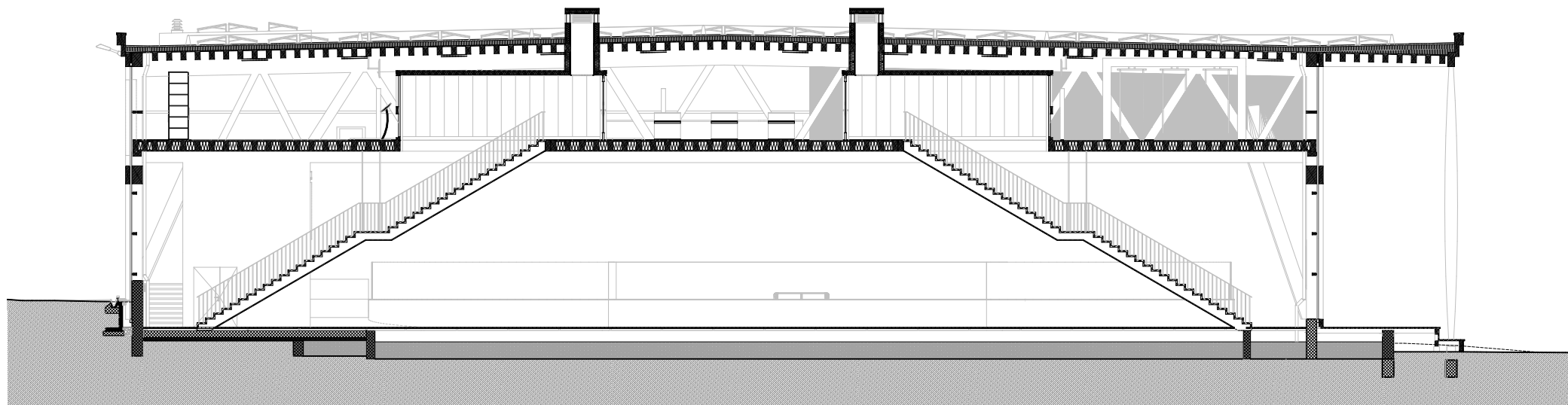
Schnitt A-A
