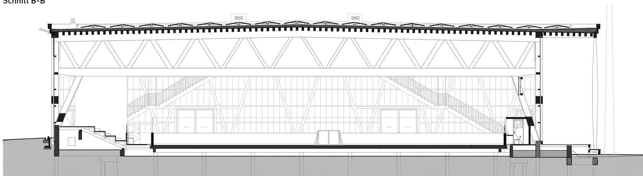
Schnitt C-C
