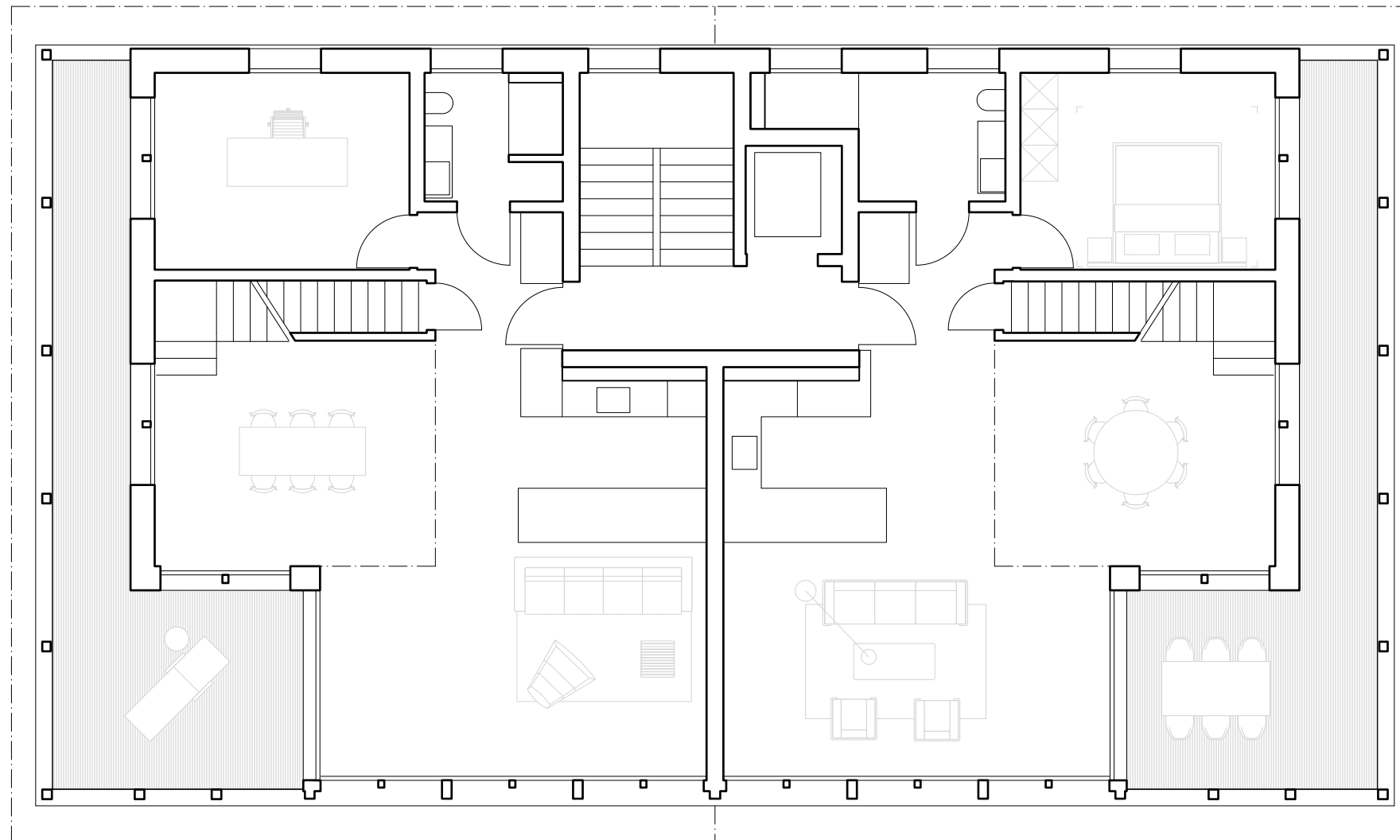
Grundriss Obergeschoss 1:100
