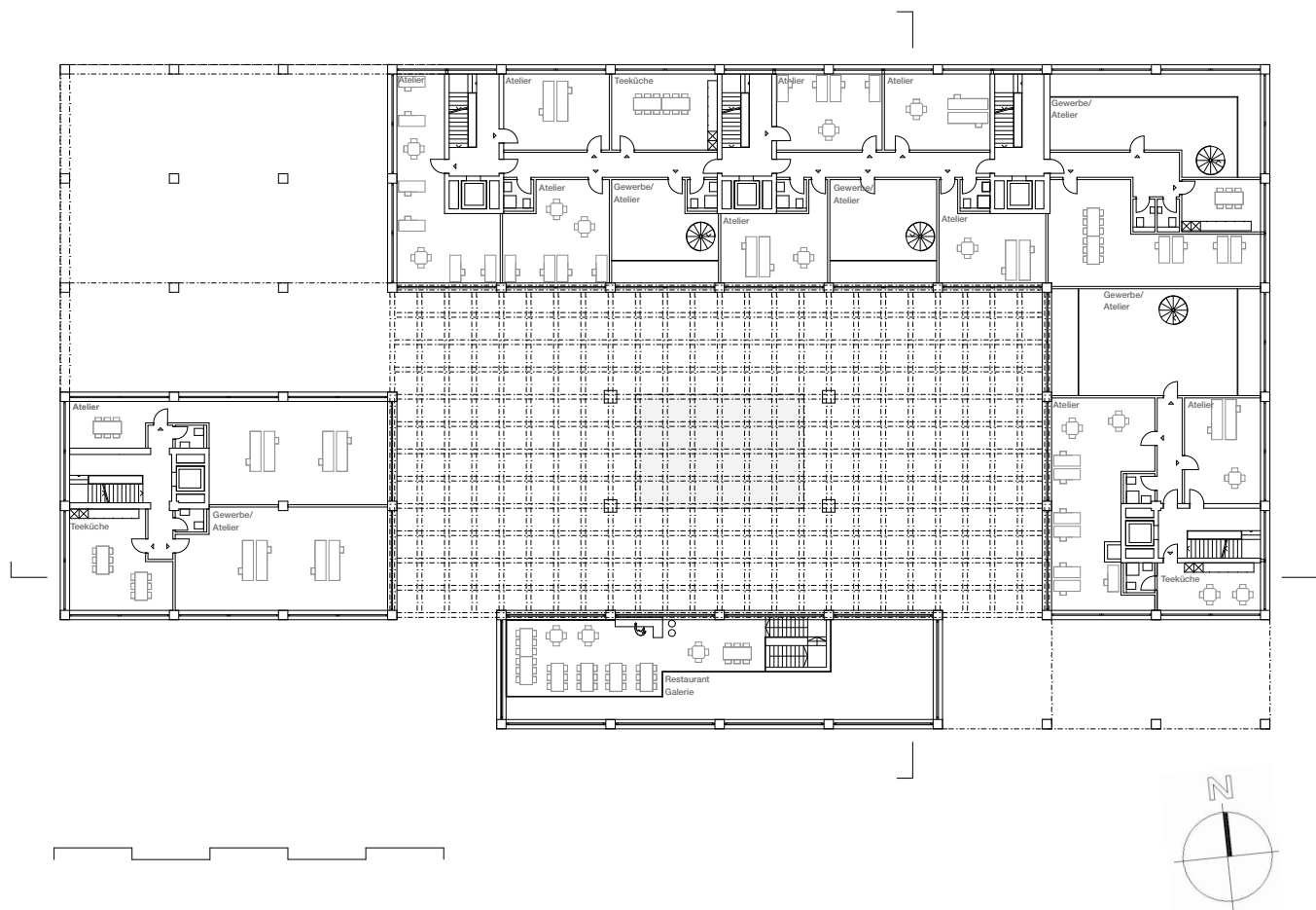
1.Obergeschoss 1:500 – Gewerbe und Atelier
