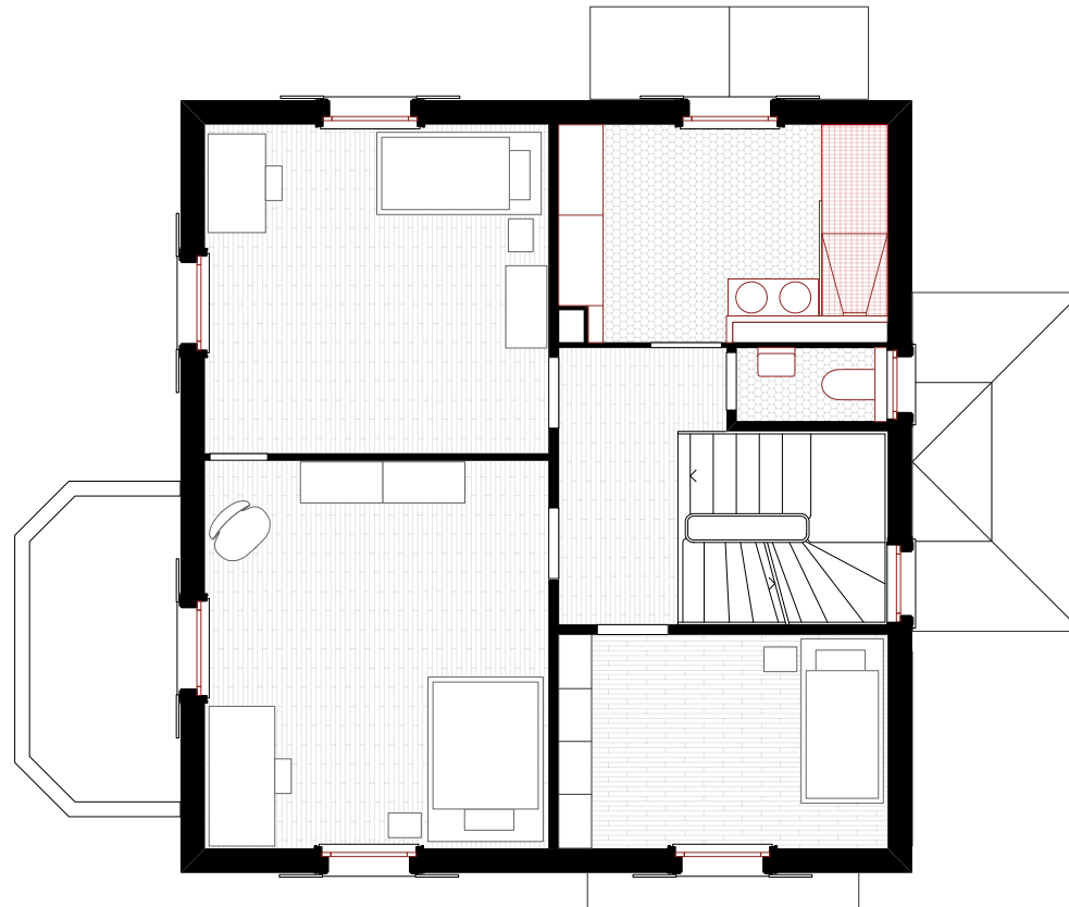
1. Obergeschoss 1:100
