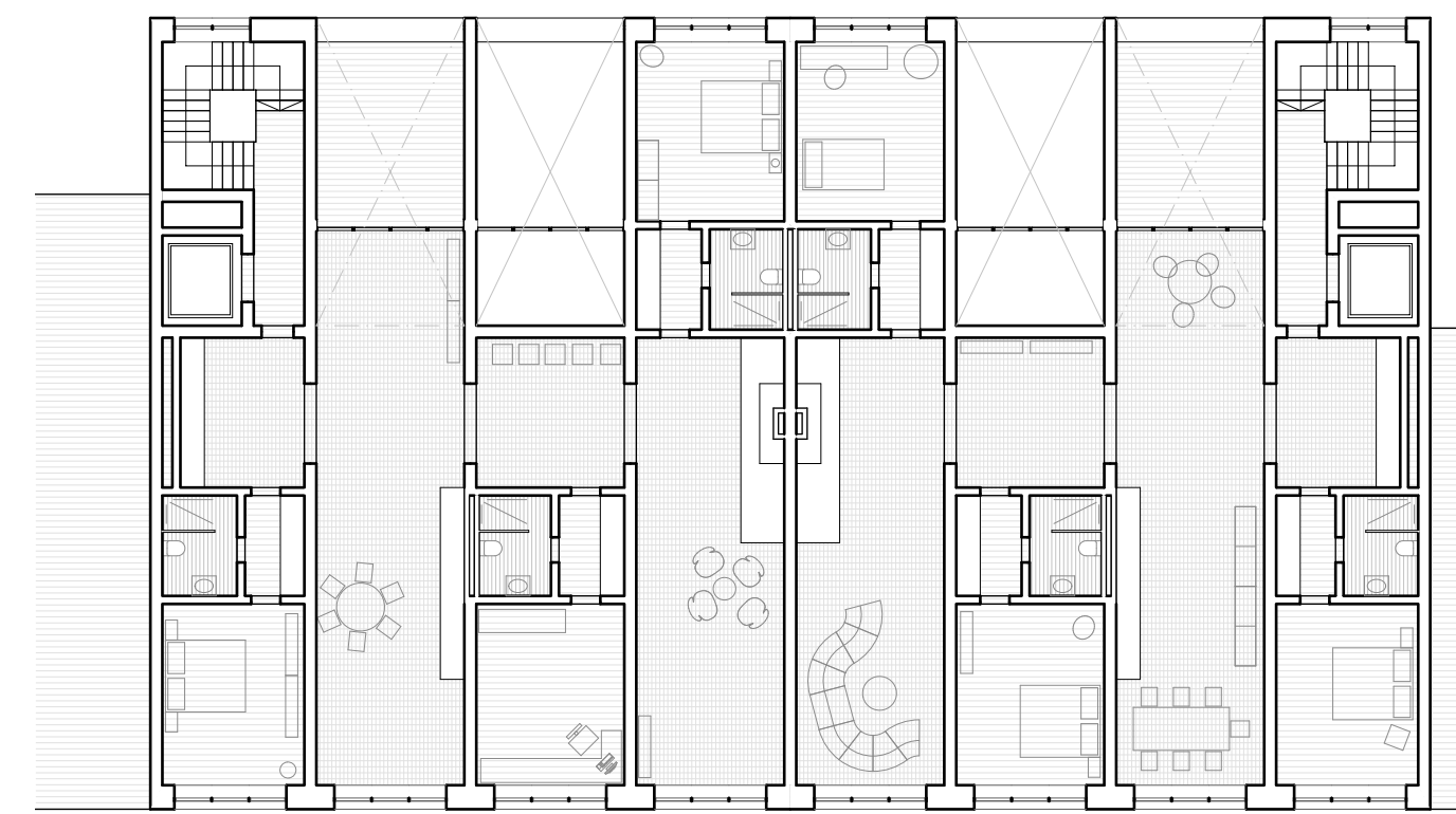
9. OG 1:200
