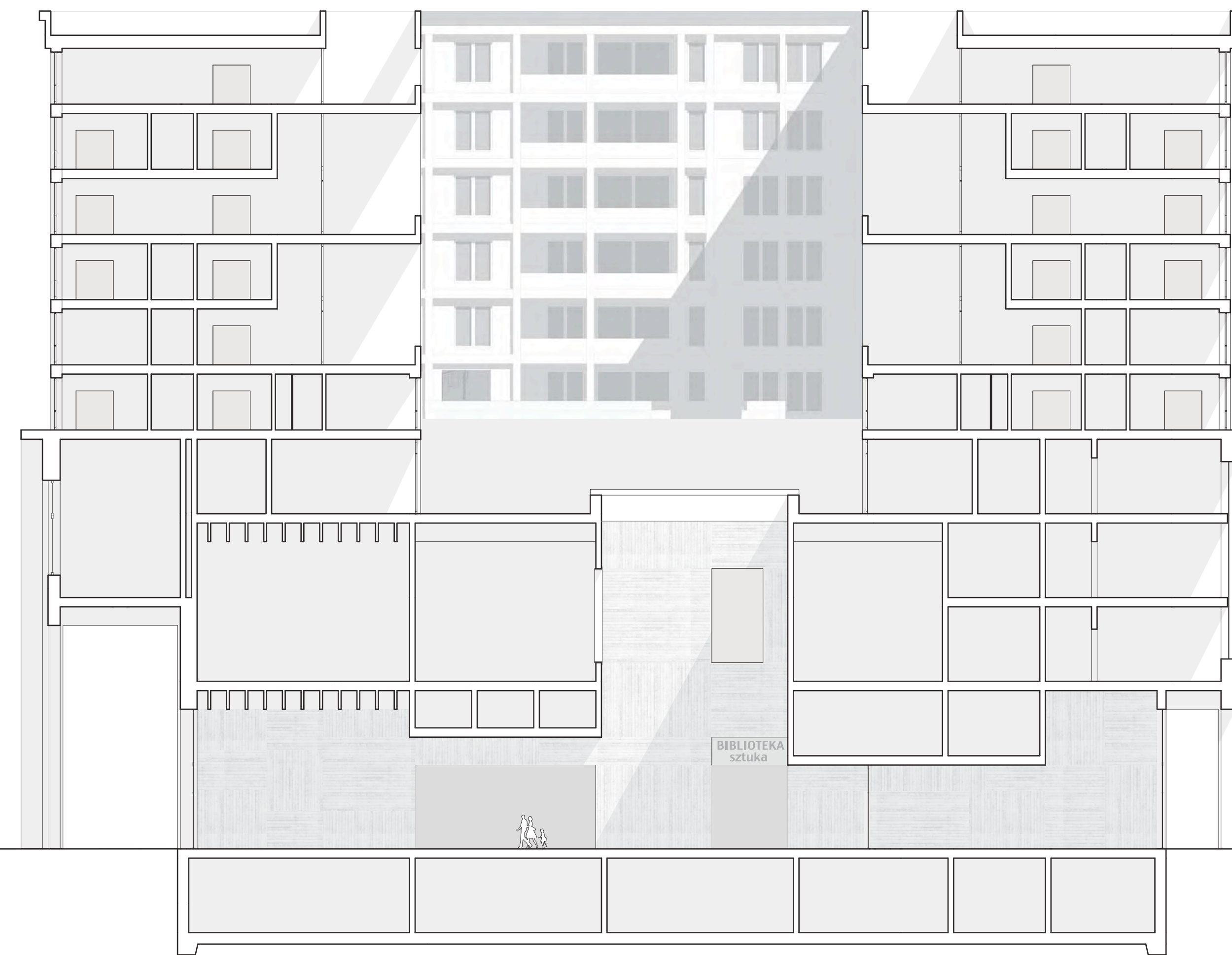
Längsschnitt 1:200
