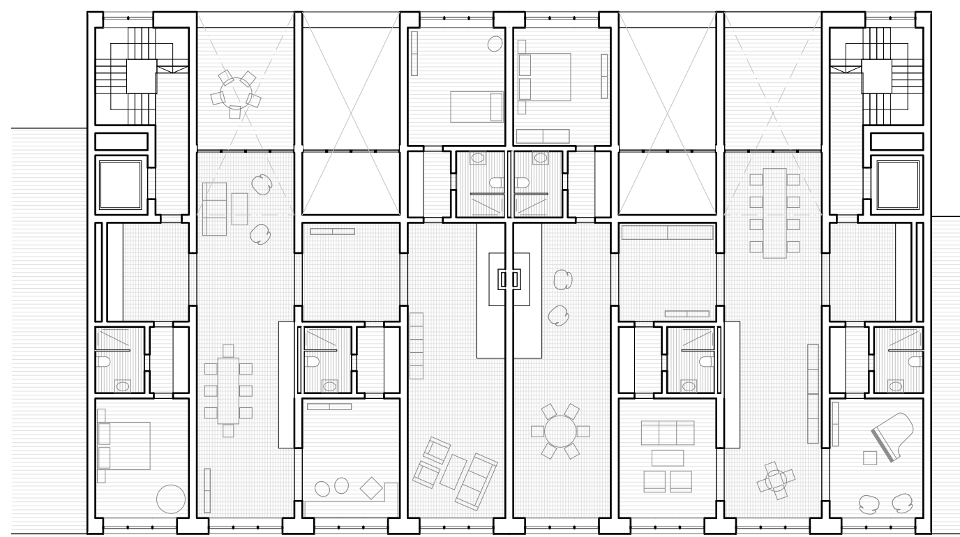
7. OG 1:200
