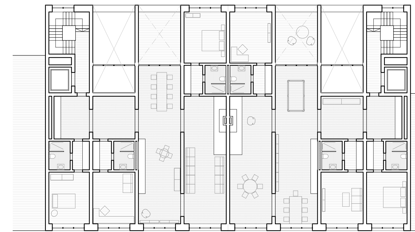
10. OG 1:200
