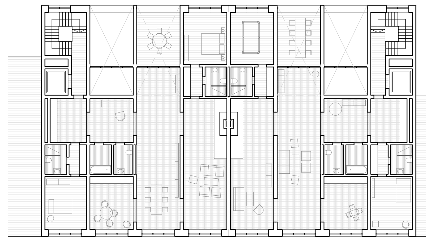
8. OG 1:200
