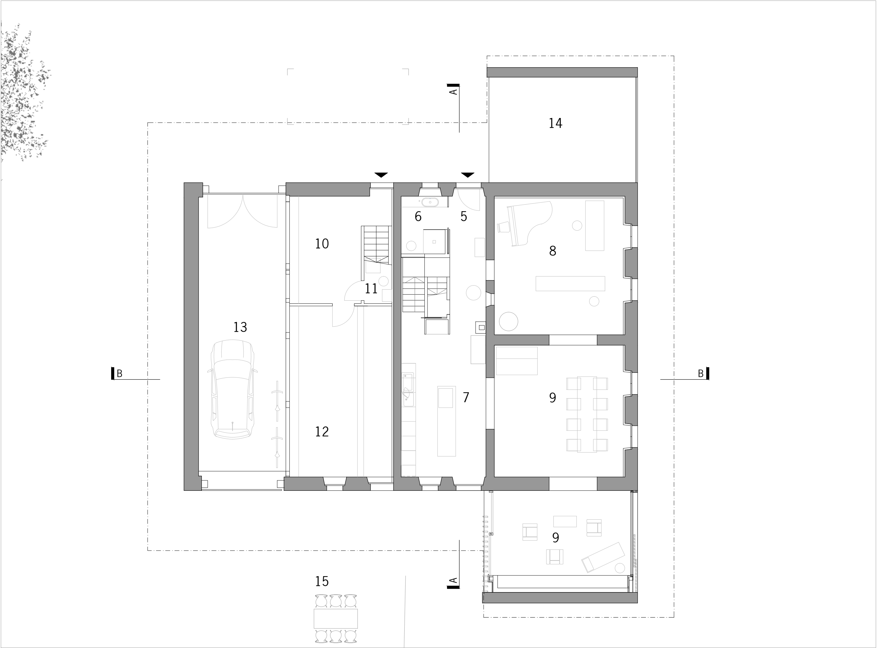
erdgeschoss/rez-de-chaussée
