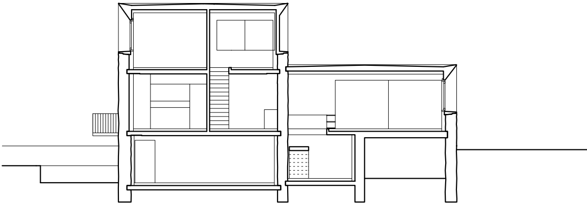
coupe longitudinale
