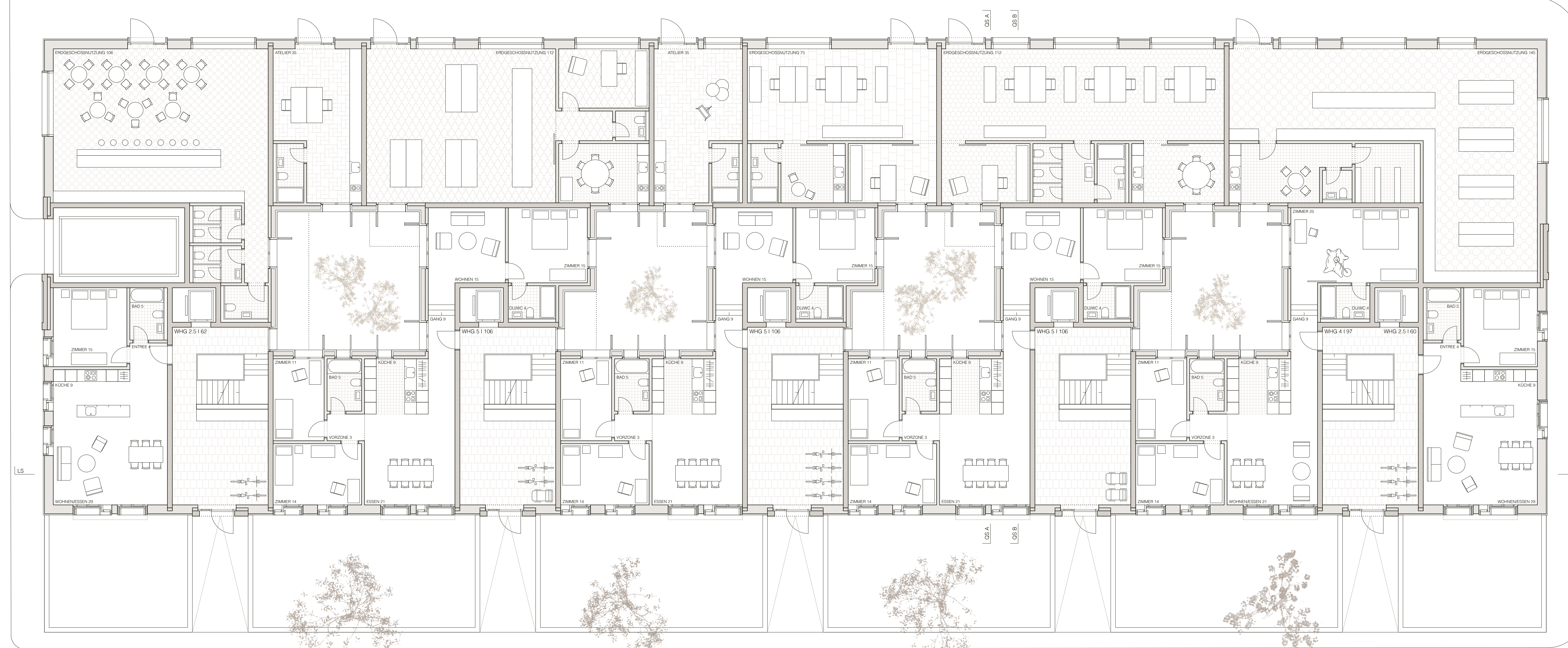
GRUNDRISS ERDGESCHOSS 1:100
