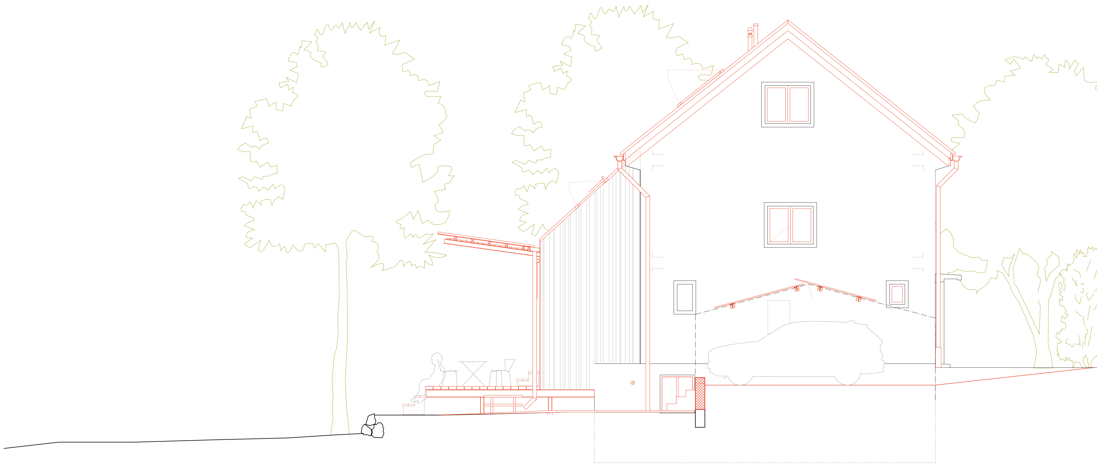
Ansicht Nord / Ost
