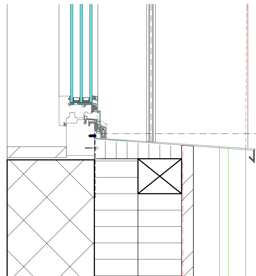
Fenster Sturz und Brüstung
