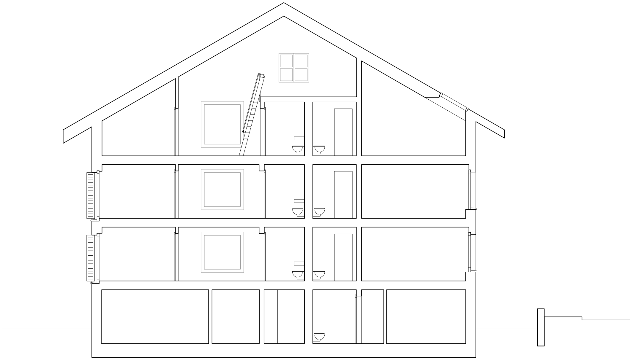
coupe transversale
