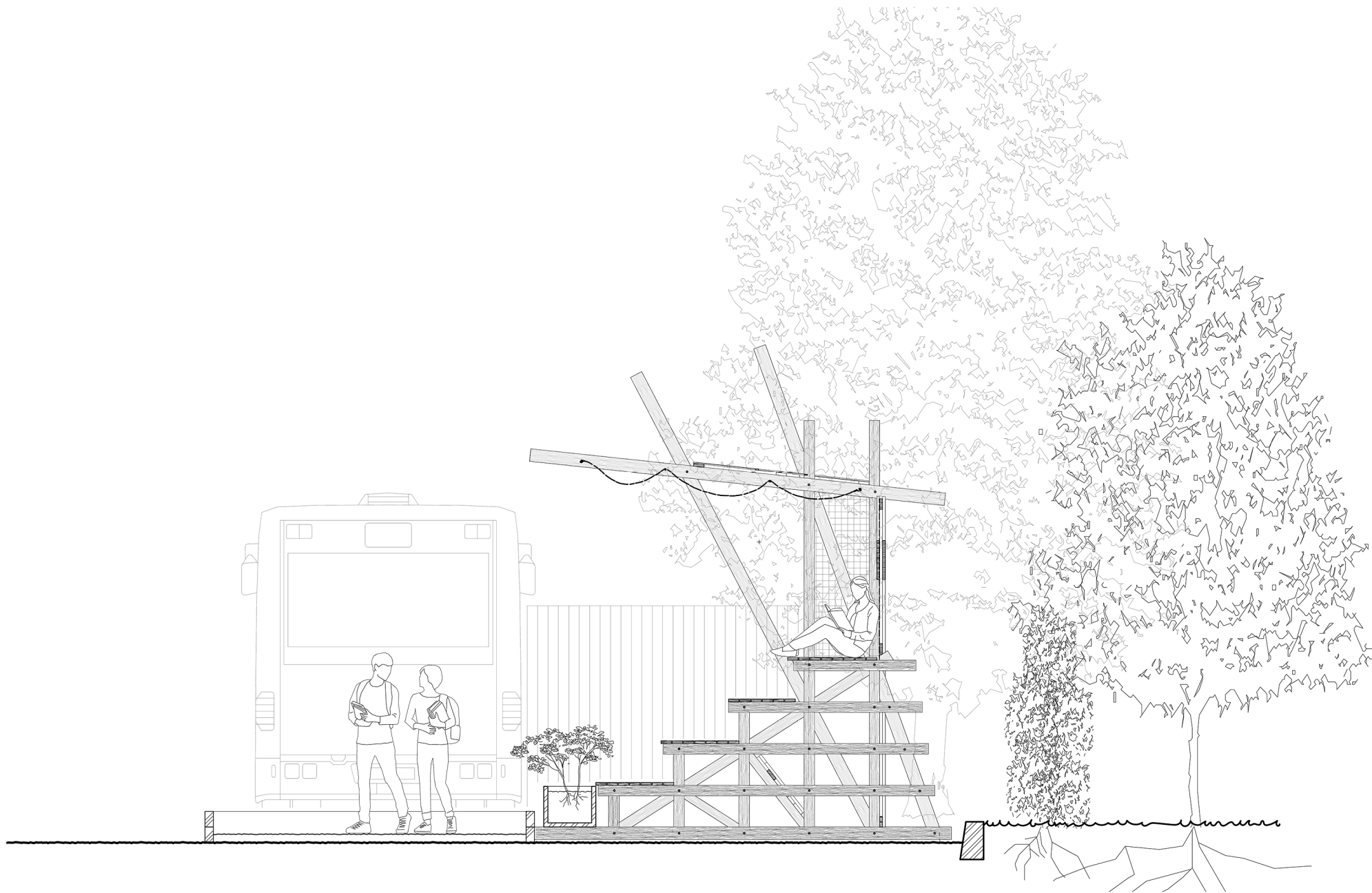
struktur «re:frame» | querschnitt | 1:50 circular time lab | standort inseli luzern | 2025
