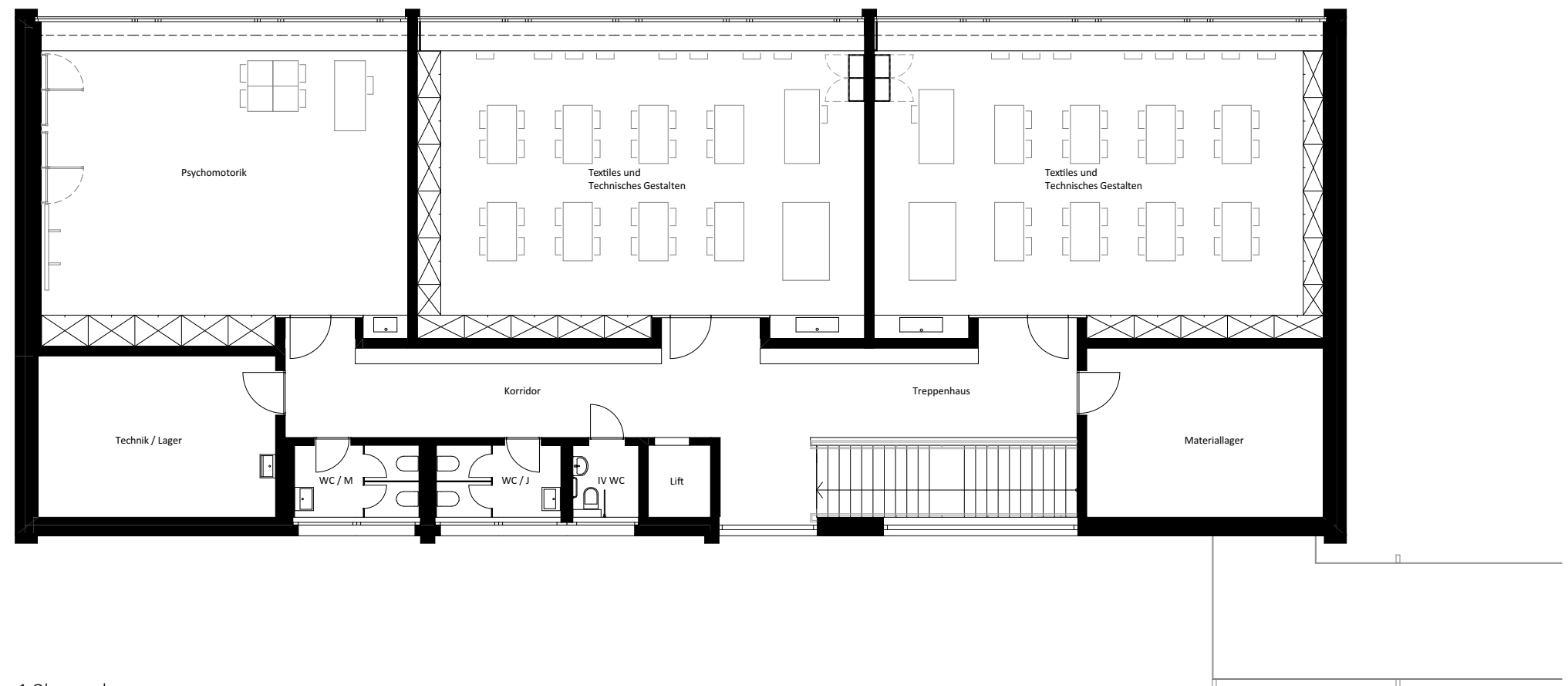
1.Obergeschoss
