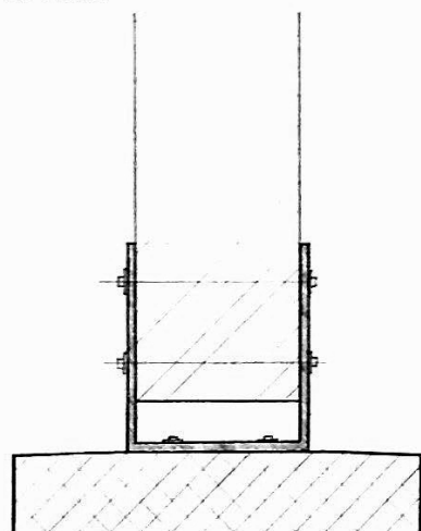
Schnitt
