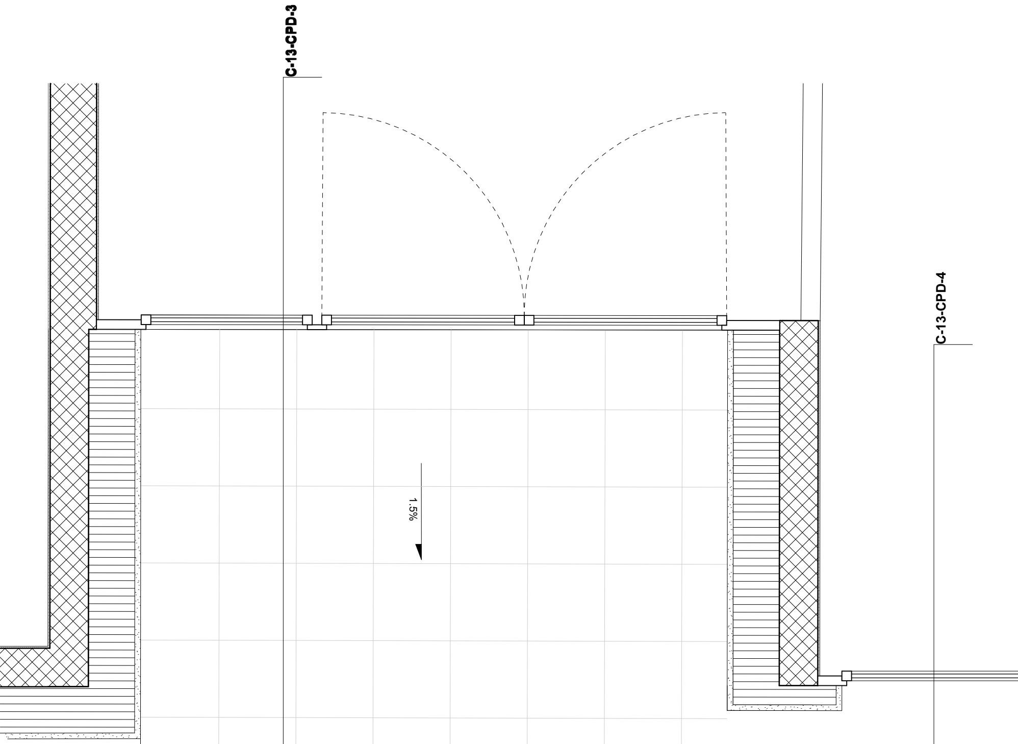
Plan loggia - rez-de-chaussée
