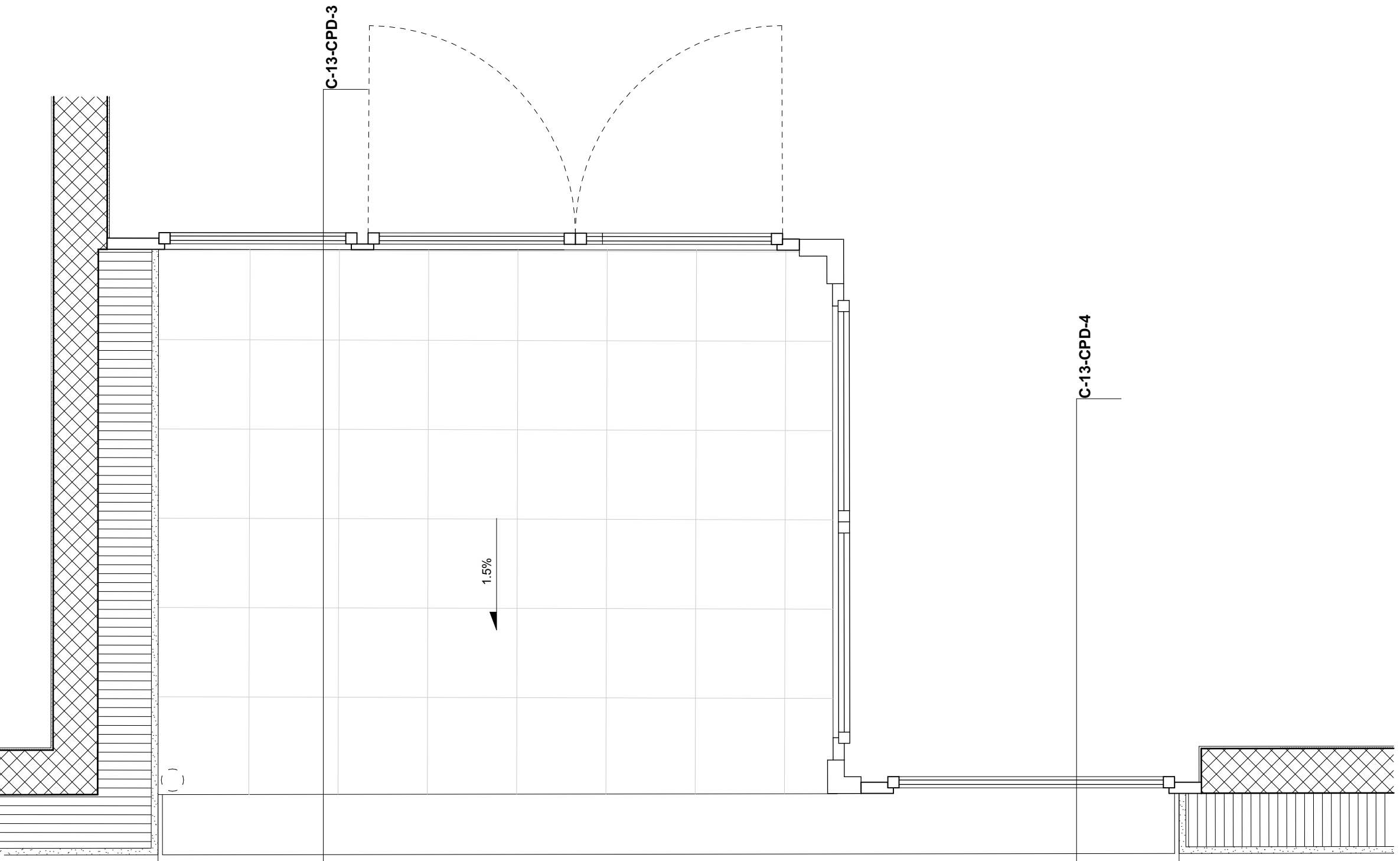
Plan loggia - 2ème étage
