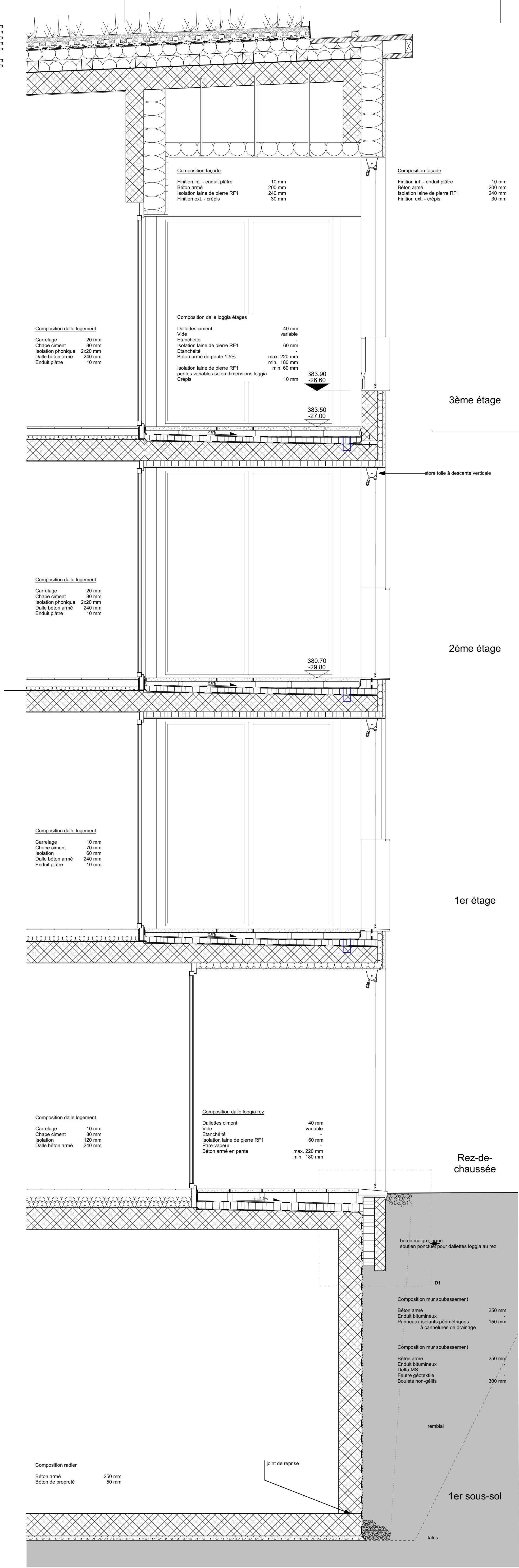
Coupe C-13-CPD-3
