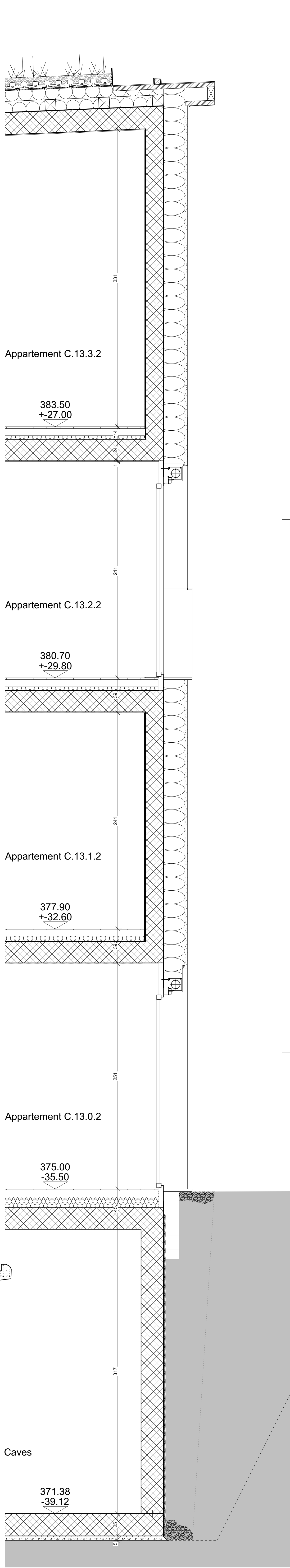
Coupe C-13-CPD-4
