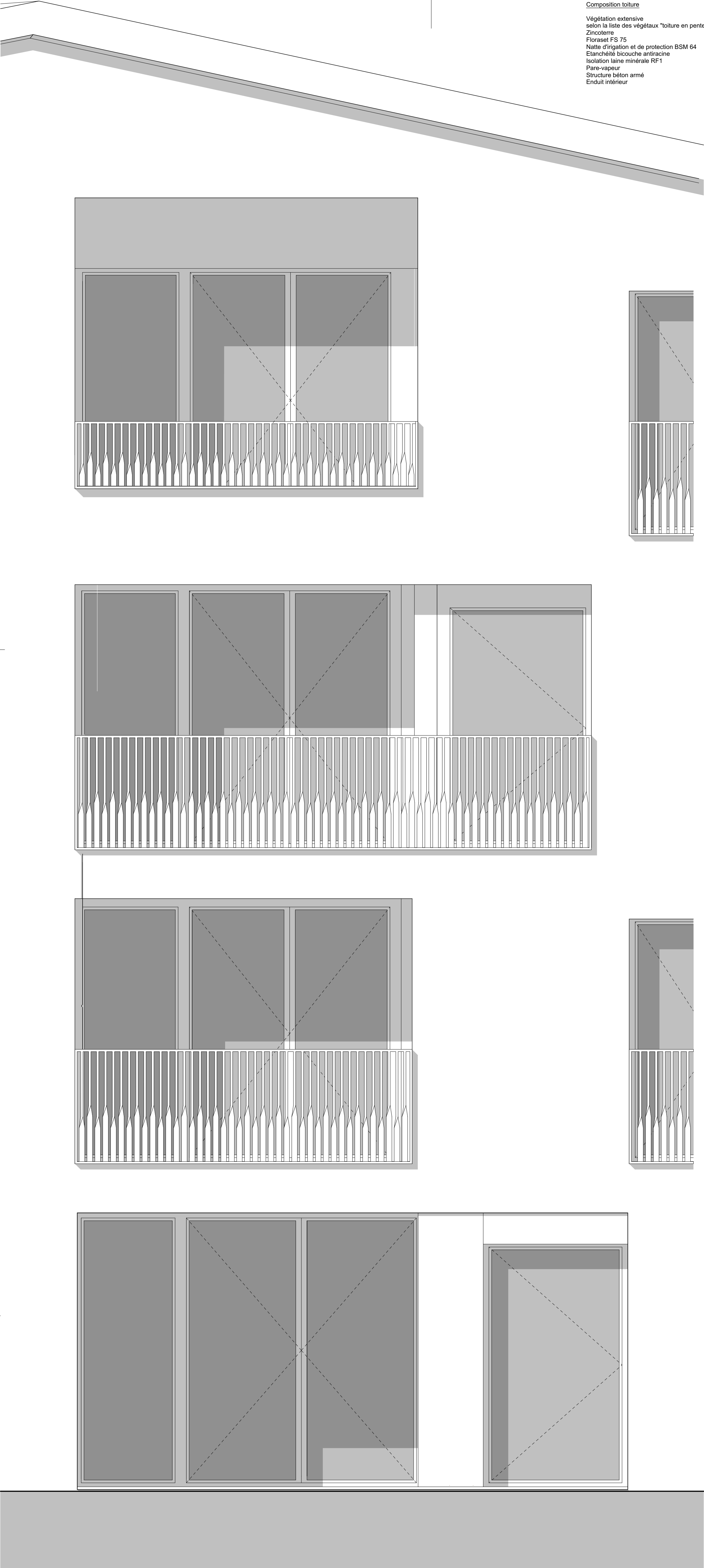
Façade sud
