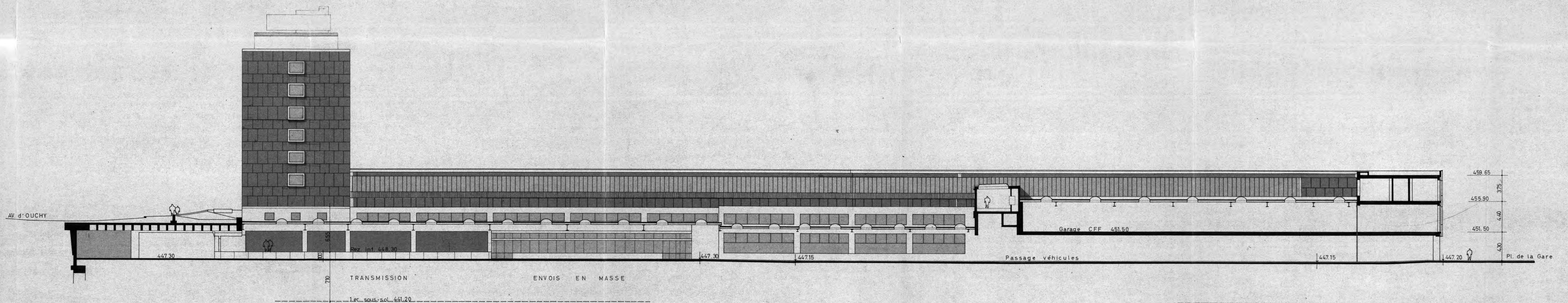
FACADE NORD ET COUPE SUR PASSAGE VEHICULES
