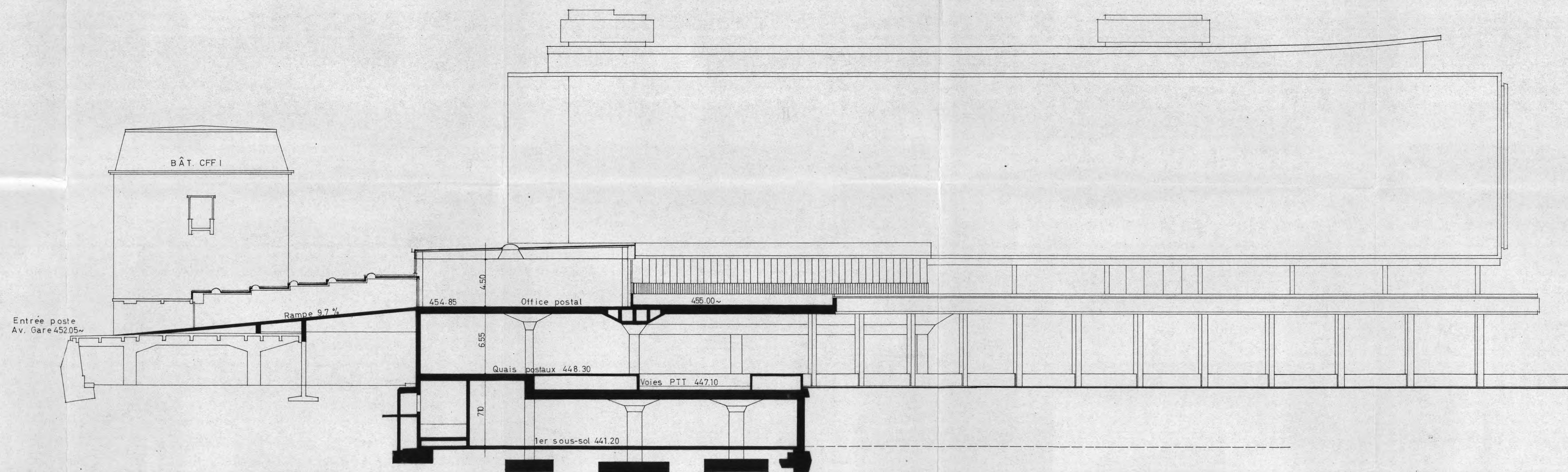
COUPE SUR ENTREE OFFICE POSTAL
