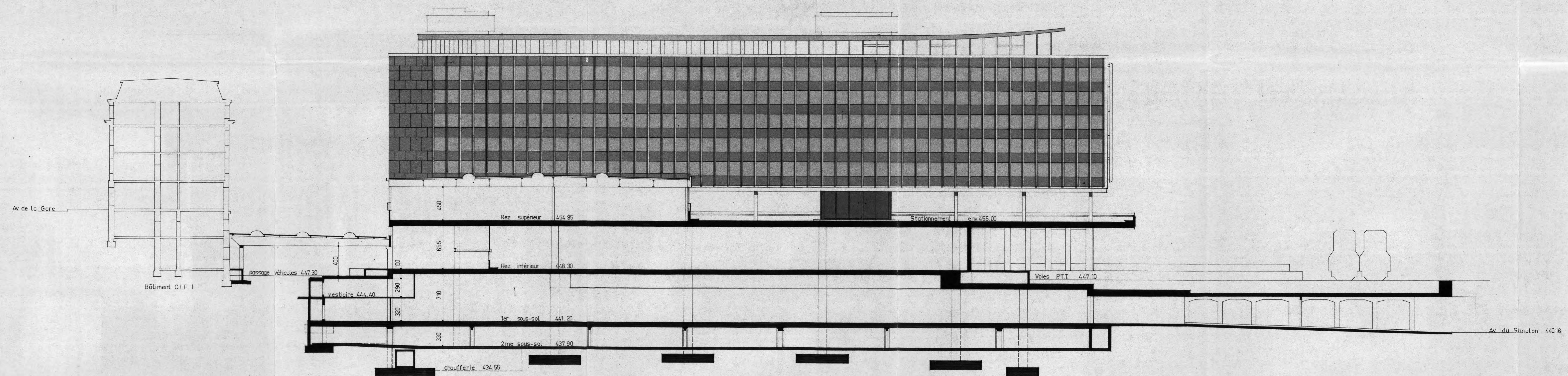
FACADE OUEST ET COUPE LONGITUDINALE SUR ENTREE AV. DU SIMPLON
