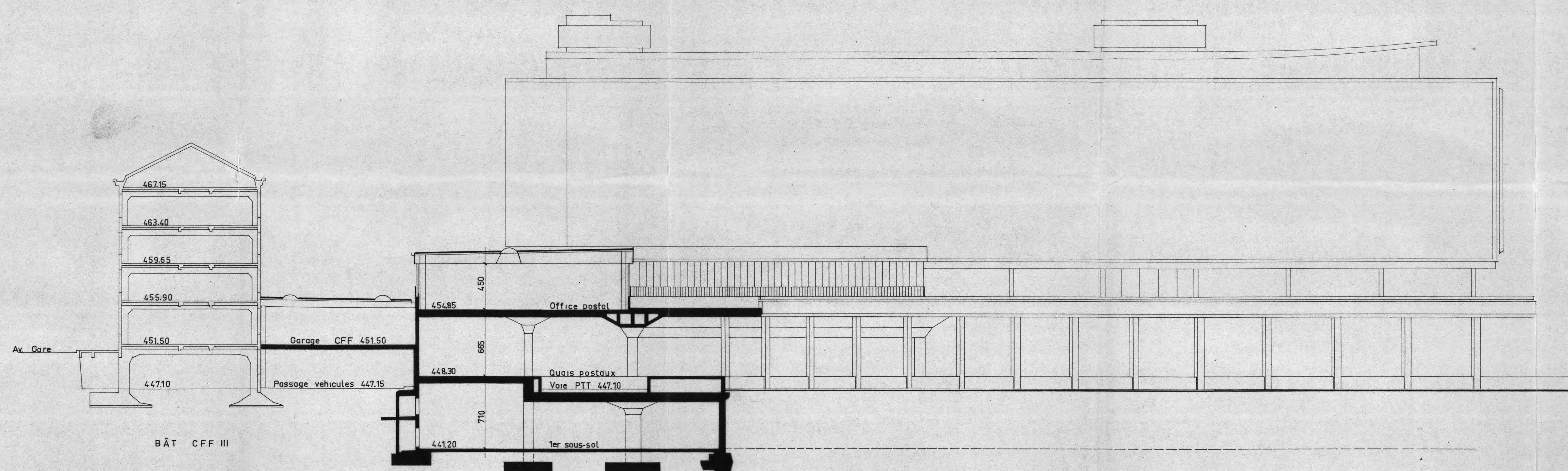
COUPE SUR GARAGE CFF ET OFFICE POSTAL
