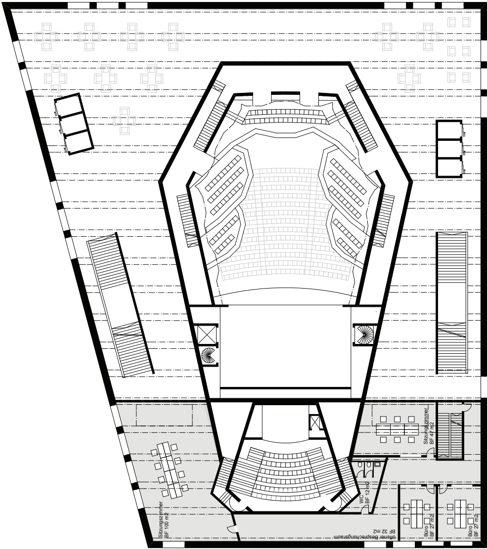
2. OG Zwischengeschoss 1:400
