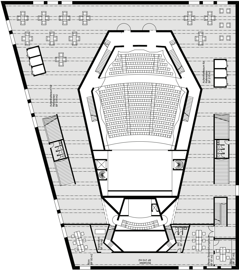
2. Obergeschoss 1:400
