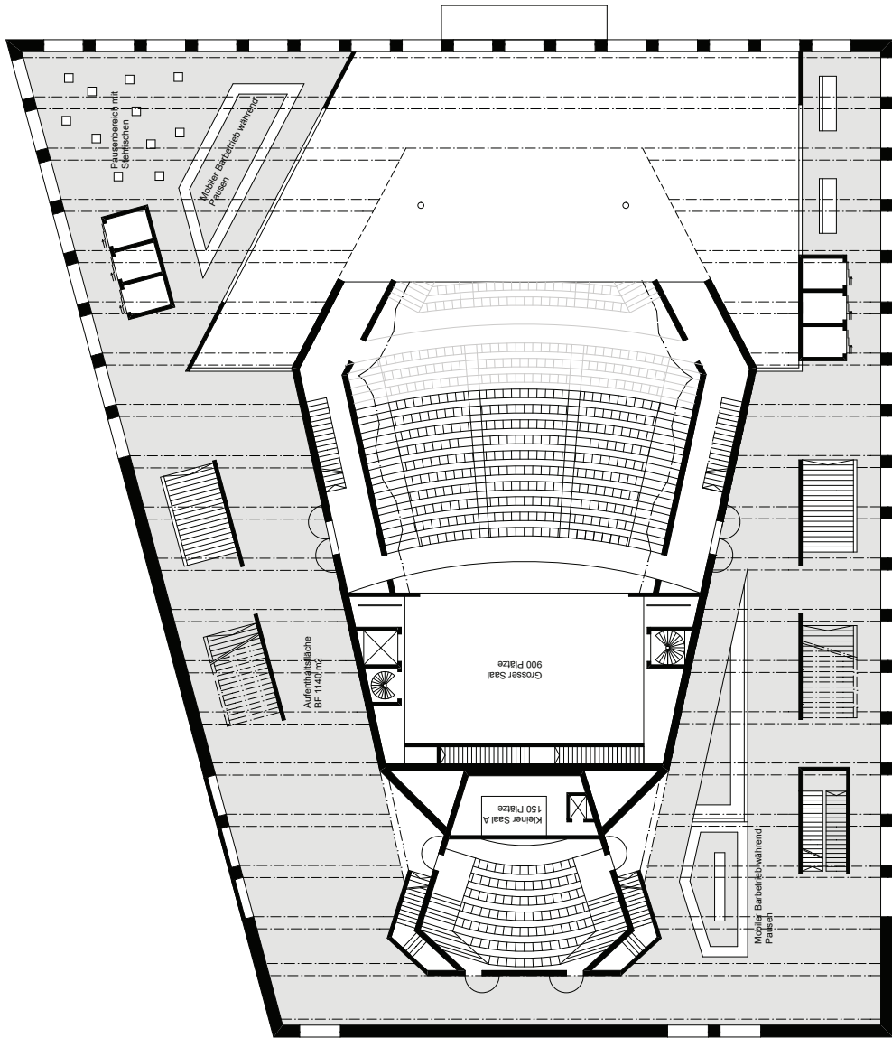
1. Obergeschoss 1:400
