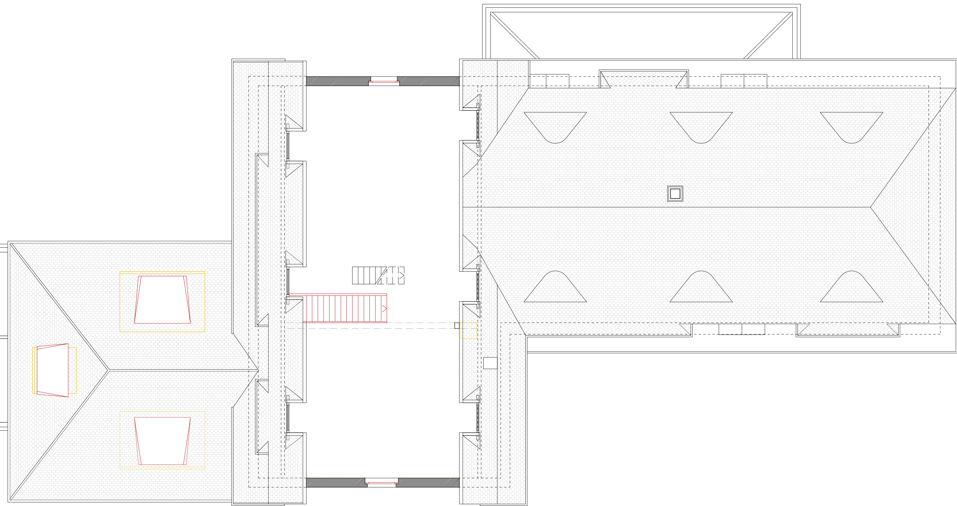
Grundriss 2. DG
