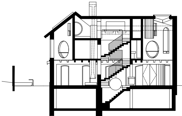
Längsschnitt | Coupe longitudinale
