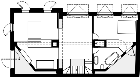
1. Obergeschoss | 1 er étage
