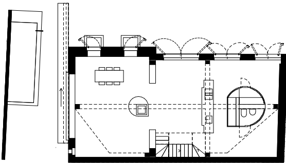
Erdgeschoss | Rez-de-chaussée
