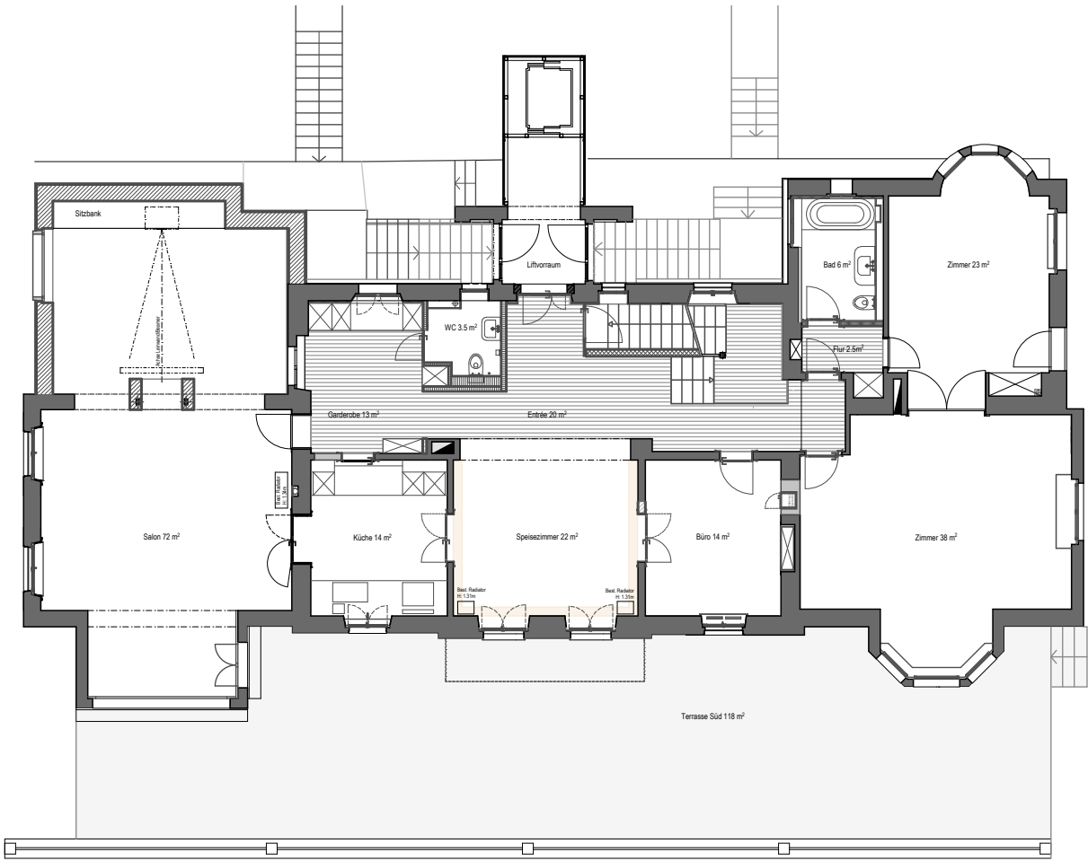
Erdgeschoss
