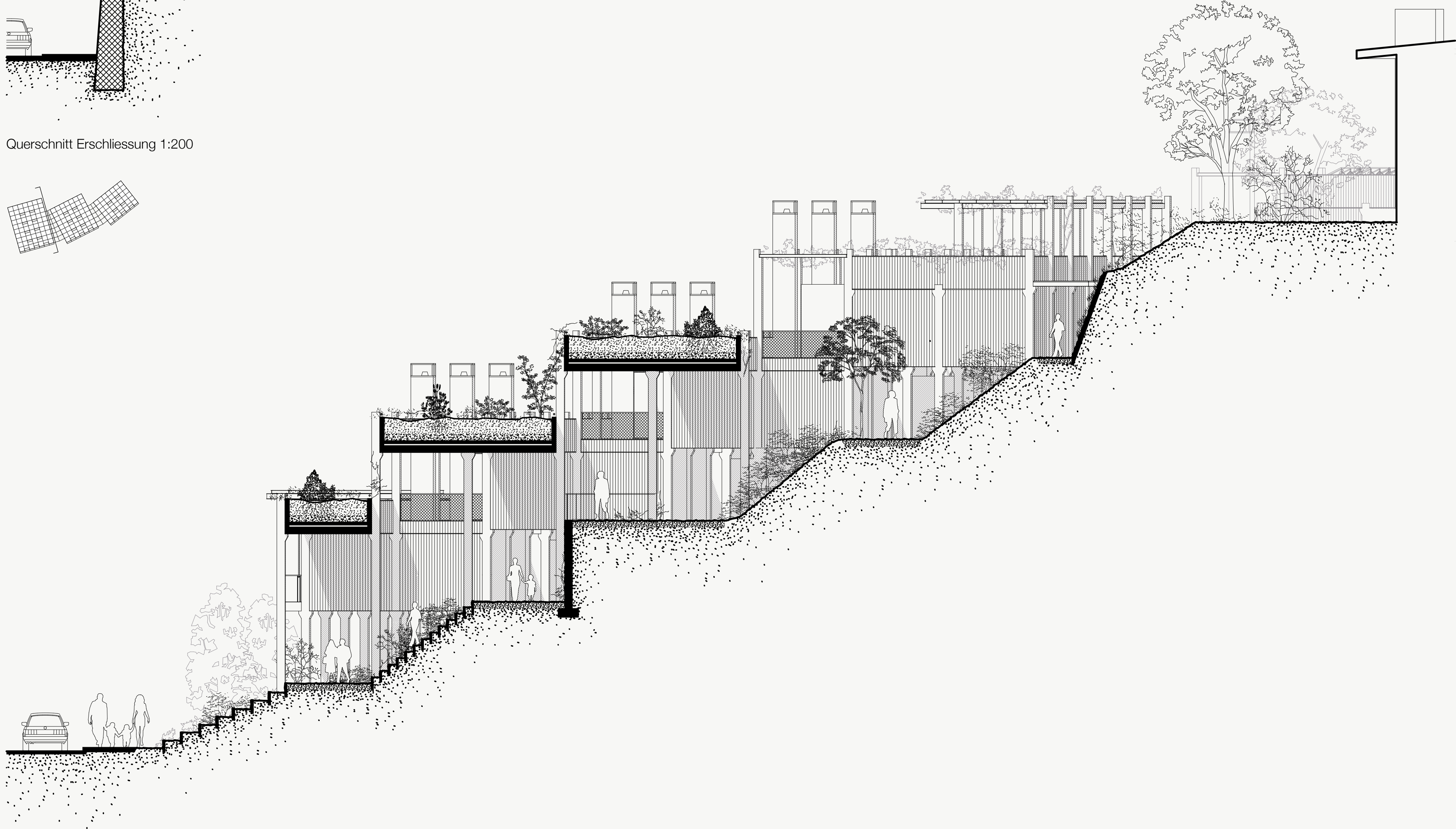
Querschnitt Erschliessung 1:200
