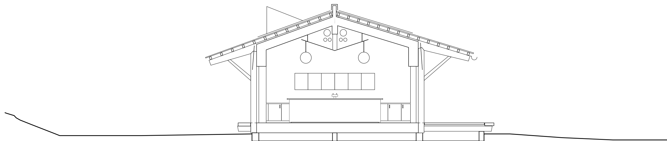
Coupe B
