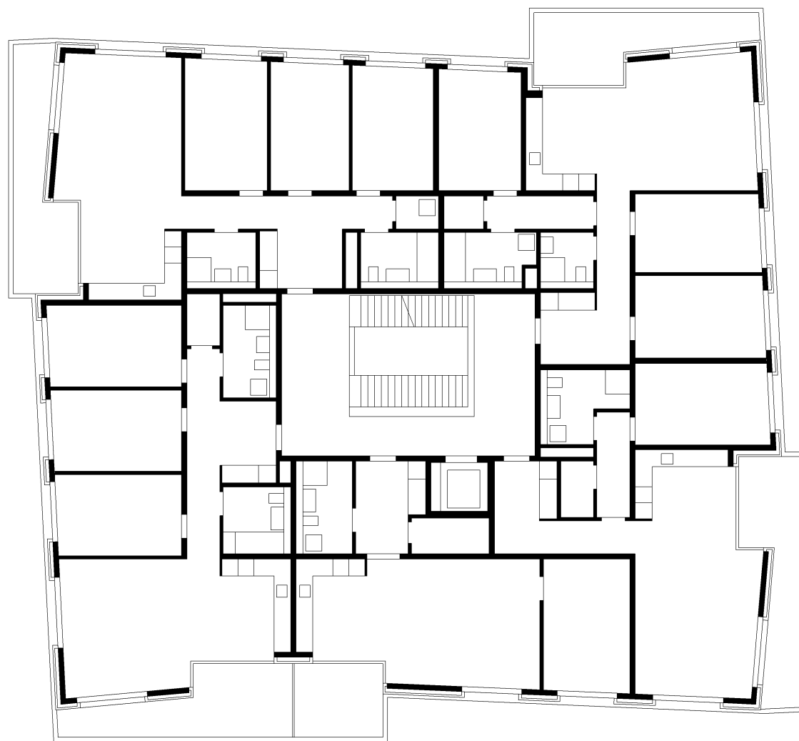
Regelgeschoss Haus L
