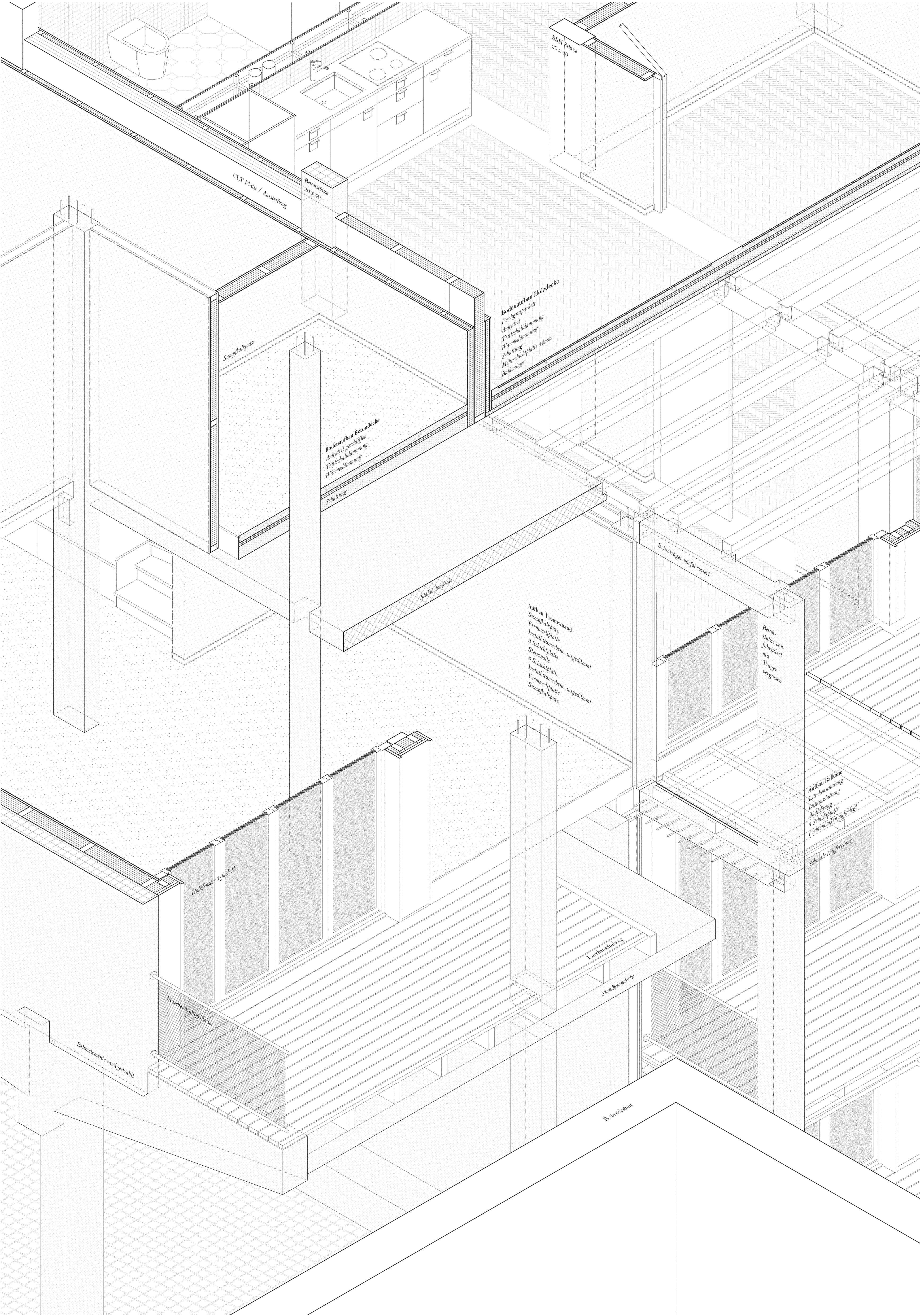
Detailaxonometrie 1_20
